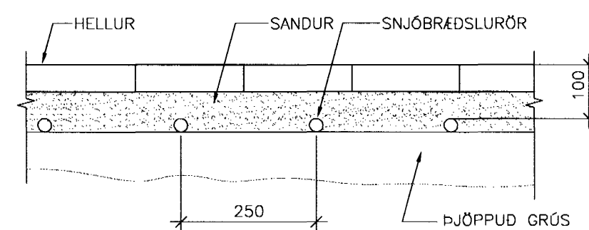
A DÆMIGERT SNID Í HELLUR, 1:10
