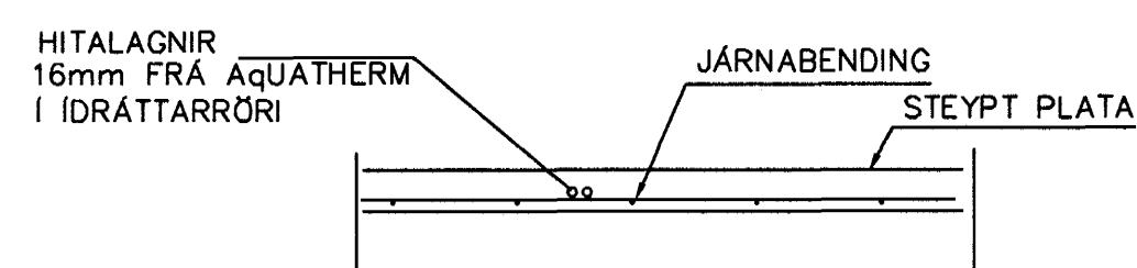
LAGNIR, SNIÐ, 1:20
