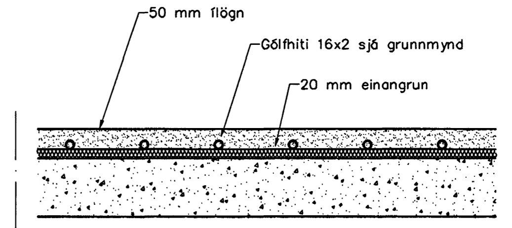
Gólfhiti, Snið í milliþötu, 1:10
