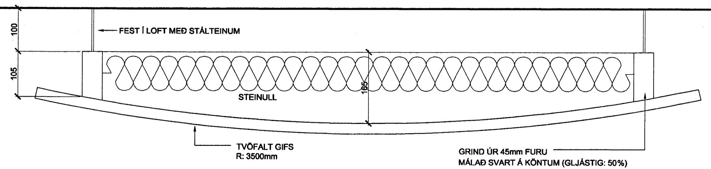
SNEIÐING - LOFTAPLATA
