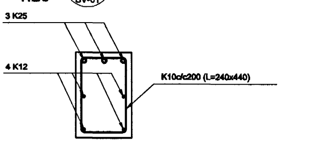
SNID M 1:20 C-B2 SV-01
