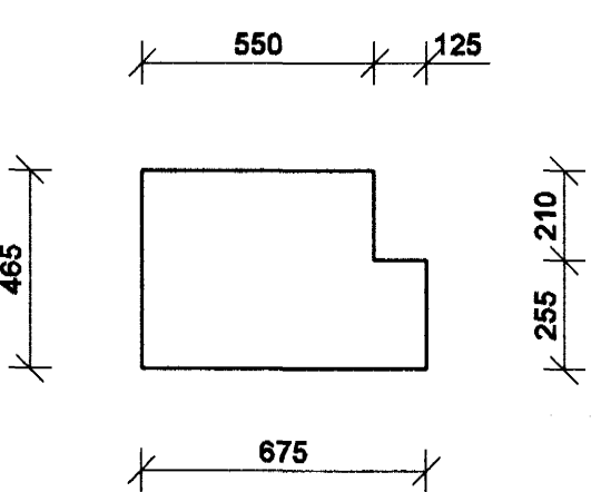
SNID L 1:20 C-B2 SV-01
