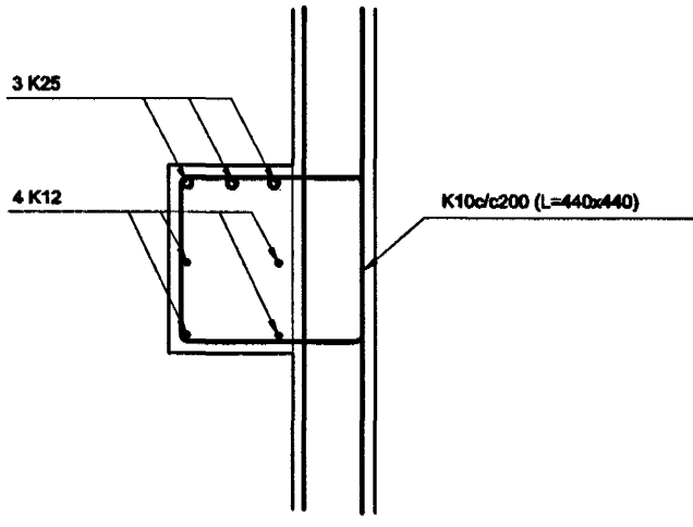
SNID M 1:20 C-B2 SV-01
