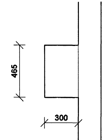
SNID M 1:20 C-B2 SV-01
