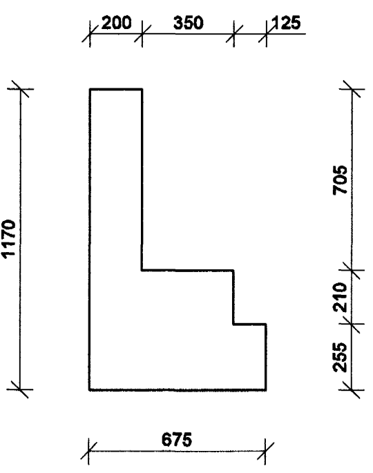
SNID K 1:20 C-B2 SV-05
