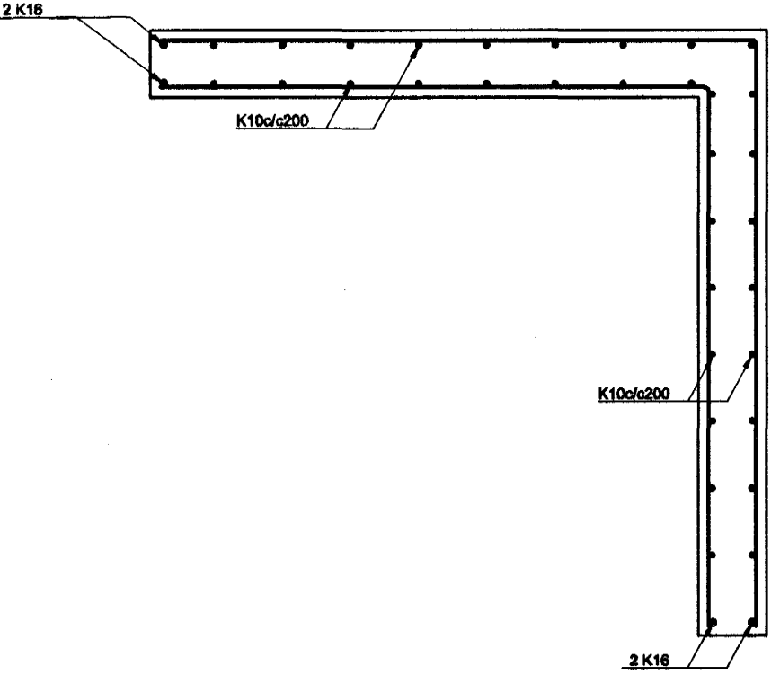
SNID K 1:20 C-B2 SV-05
