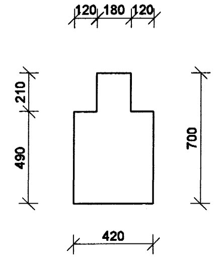
SNID B-D 1:20 C-B2 SV-07
