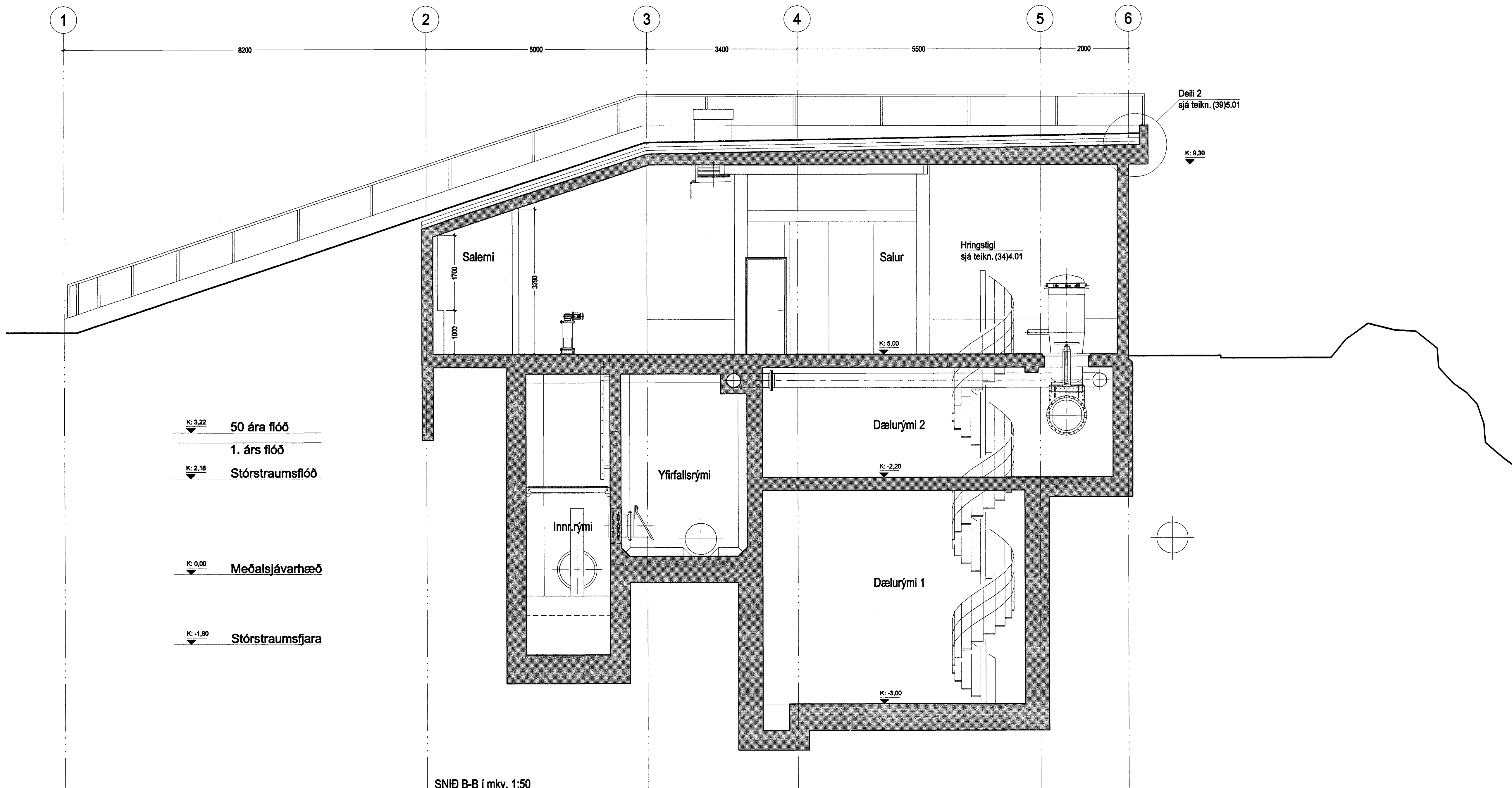
SNID B-B í mkv. 1:50
