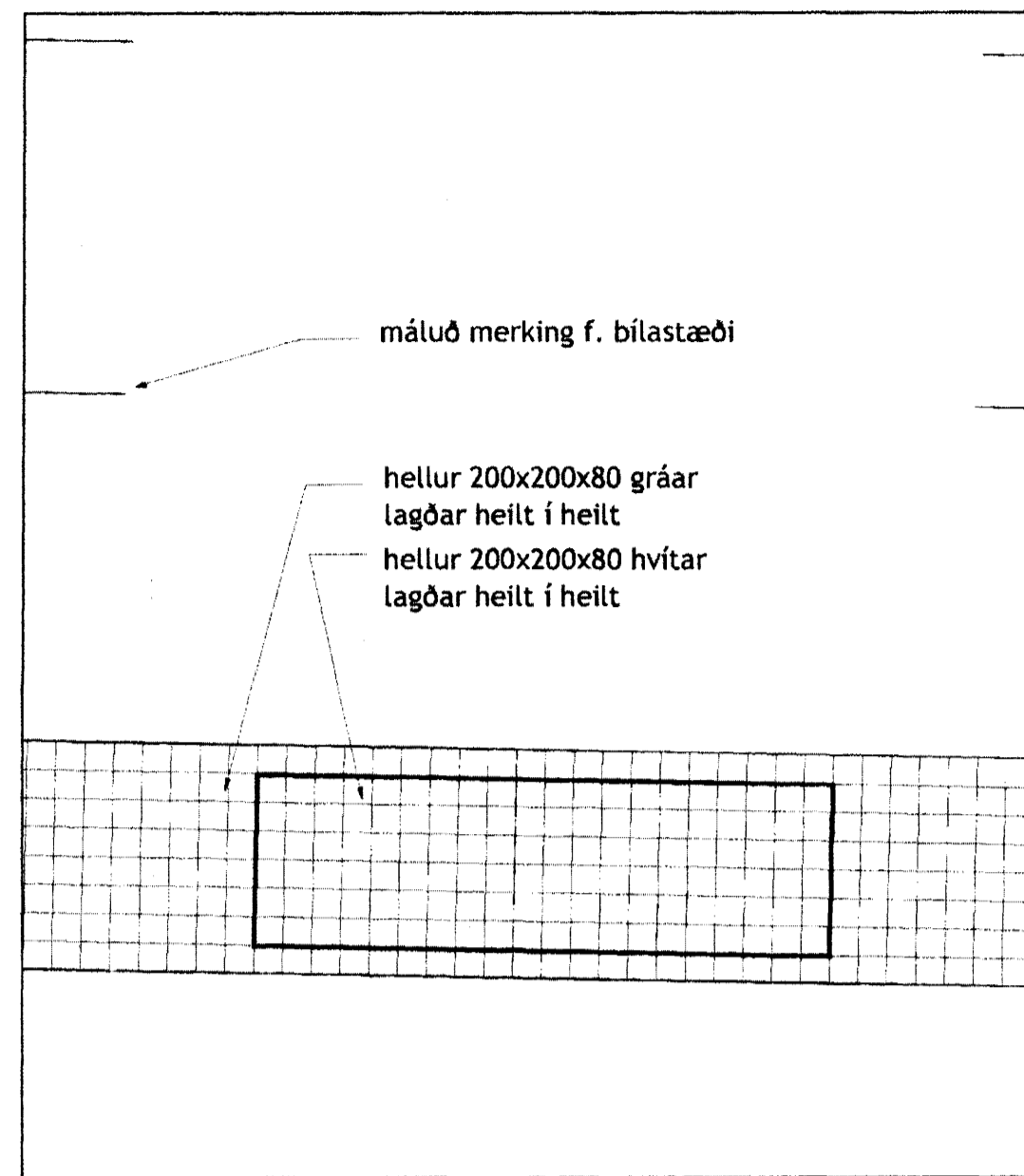
HELLULÖGN VIÐ GÖNGULEIÐ Í BÍLASTÆÐI mkv 1:50
