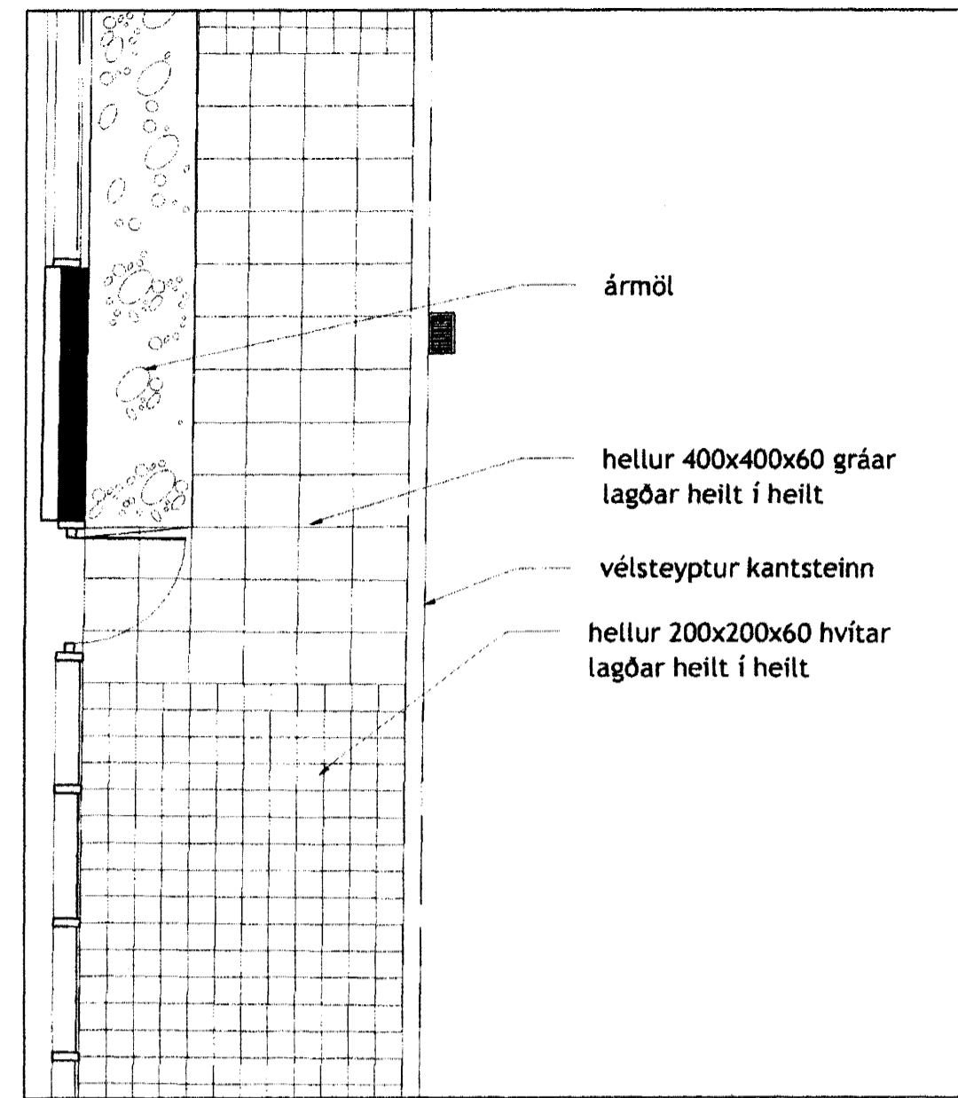
HELLULÖGN VIÐ INNGANG OG MALARBED mkv 1:50
