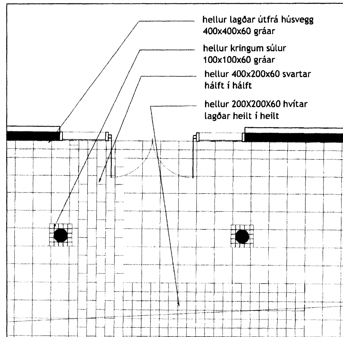
DÆMIGERÐ HELLULÖGN mkv 1:50
