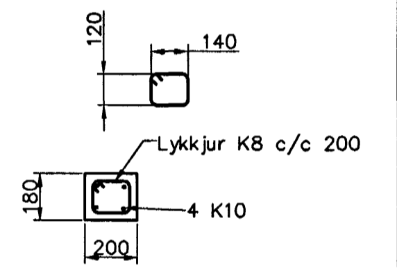
Súla S2.2 1:20
