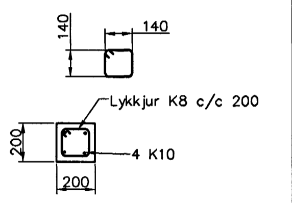
Súla S2.1 1:20
