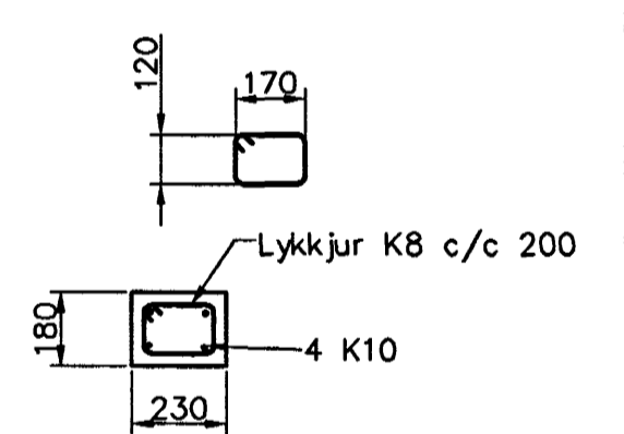
Súla S2.3 1:20
