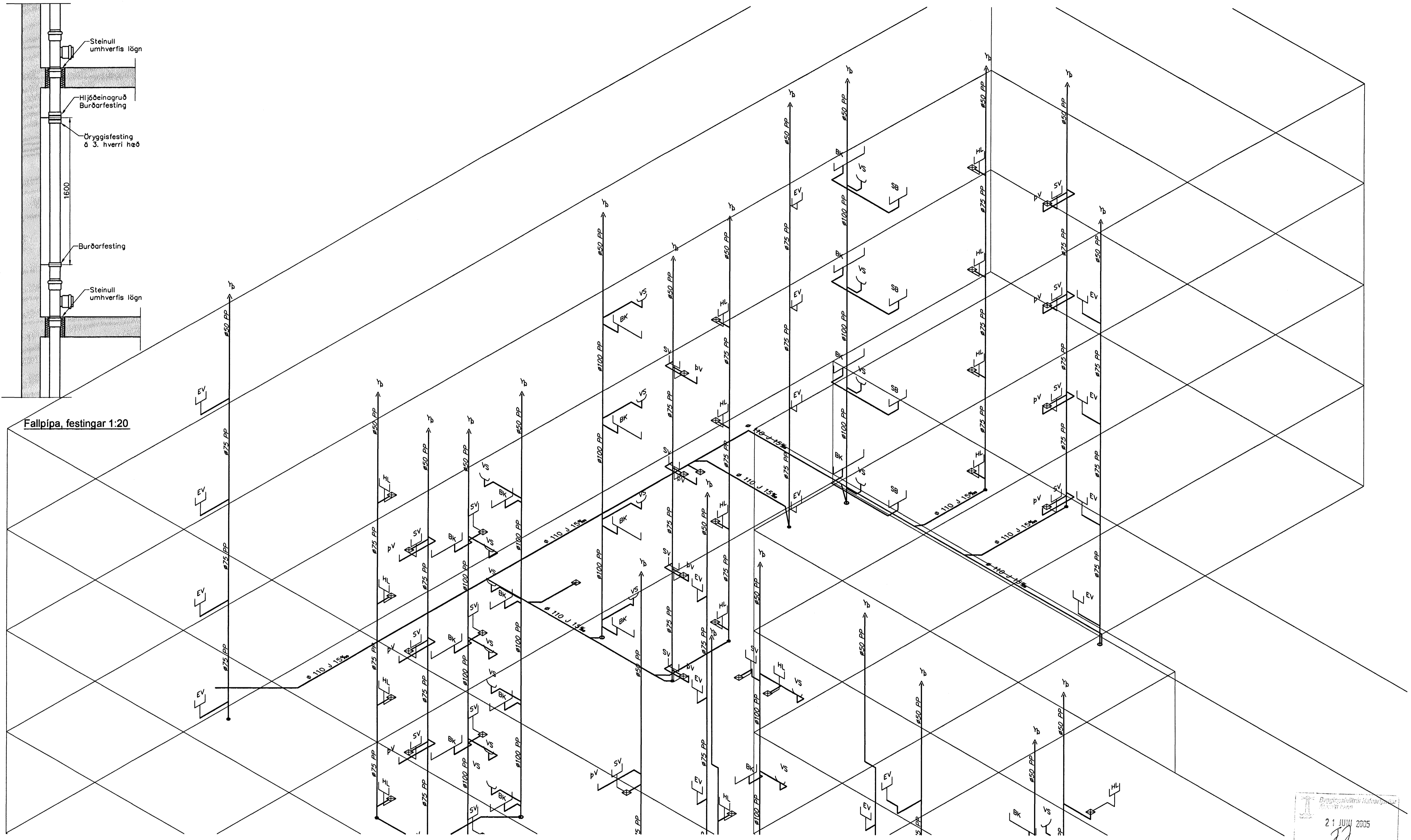
Fráveitulagnirlagnir, Rúmmynd, 1:50
