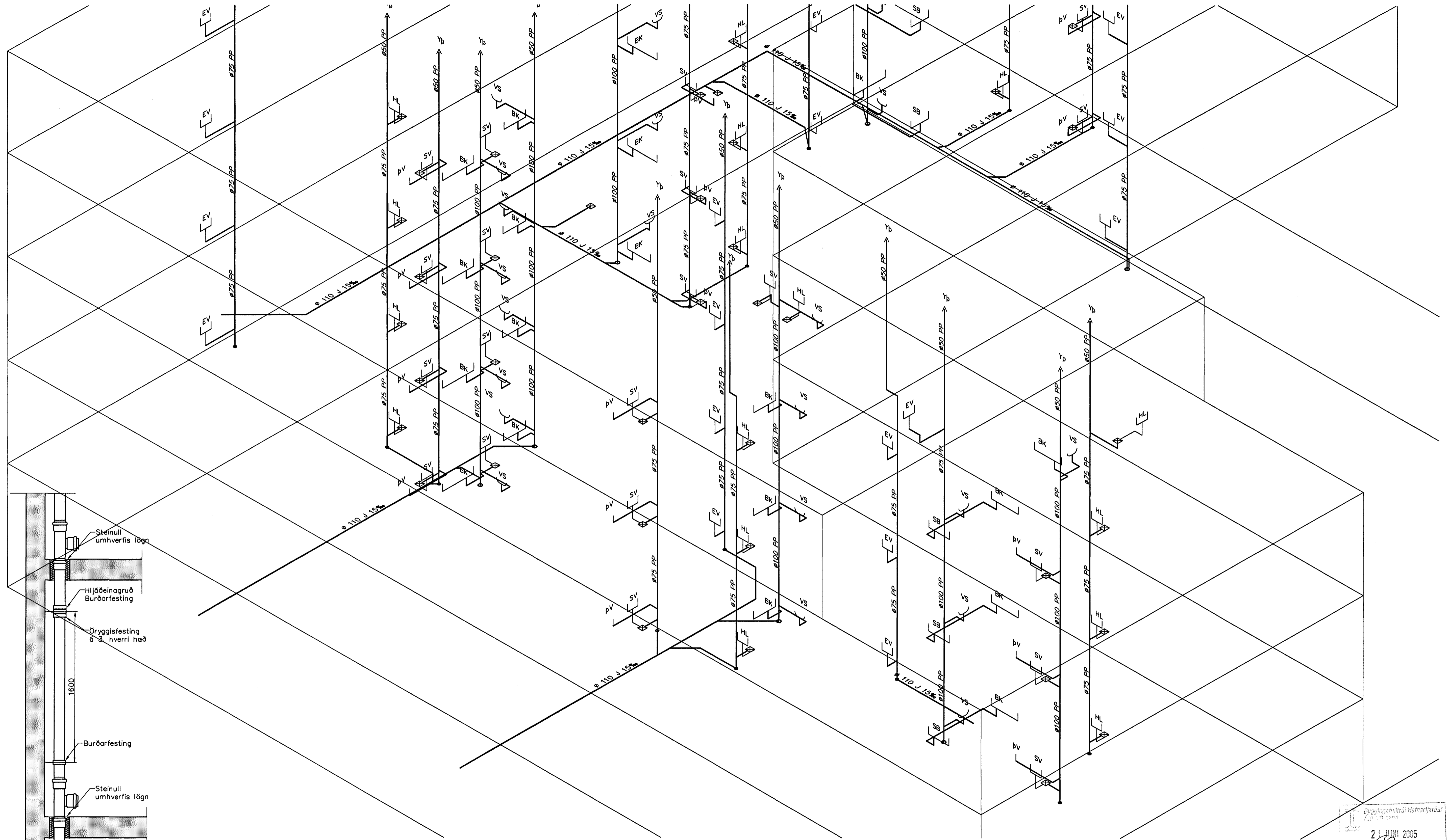
Fráveitulagnirlagnir, Rúmmynd, 1:50
