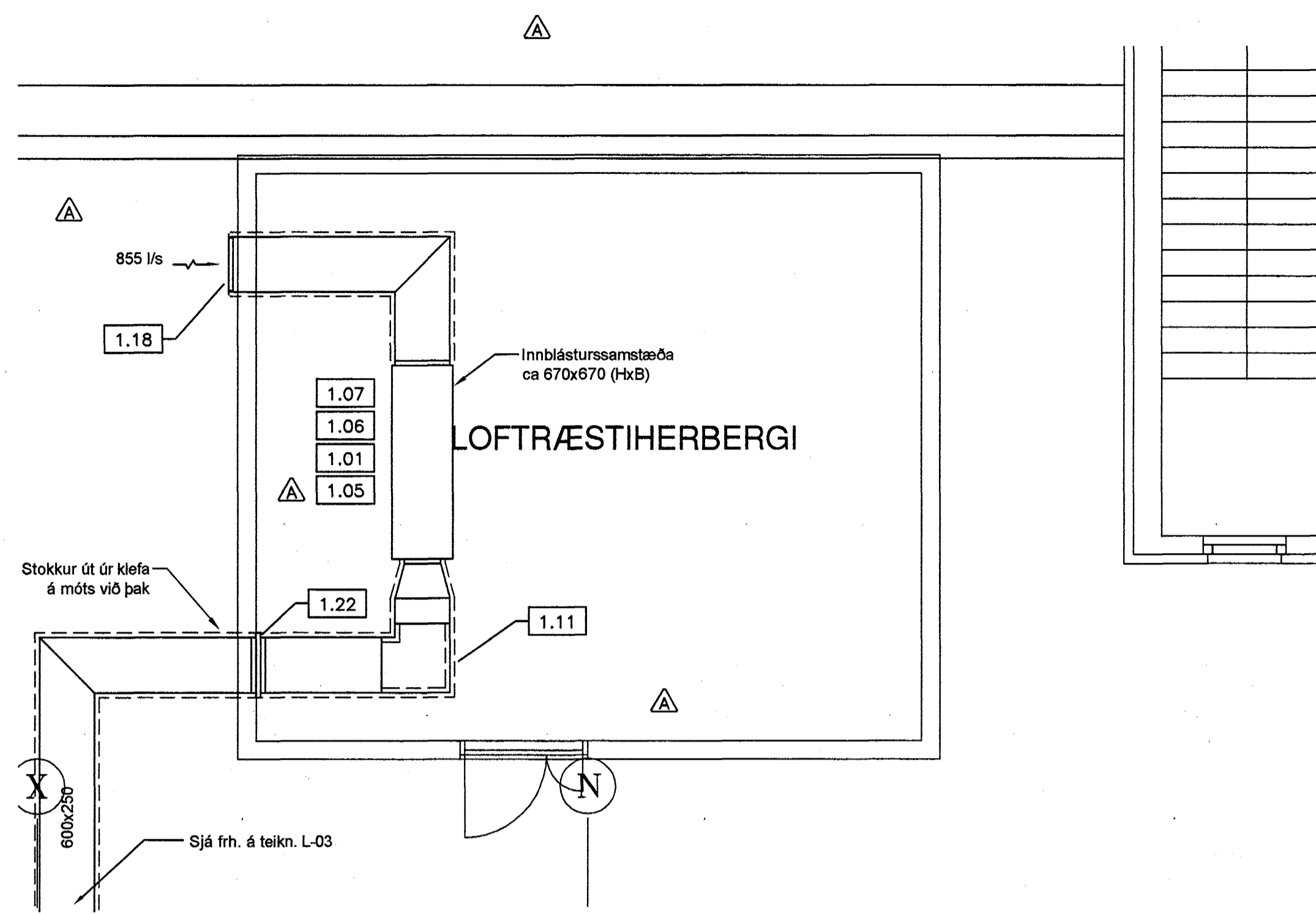
GRUNNMYND -- LOFTRÆSIKLEFI M. 1:50
