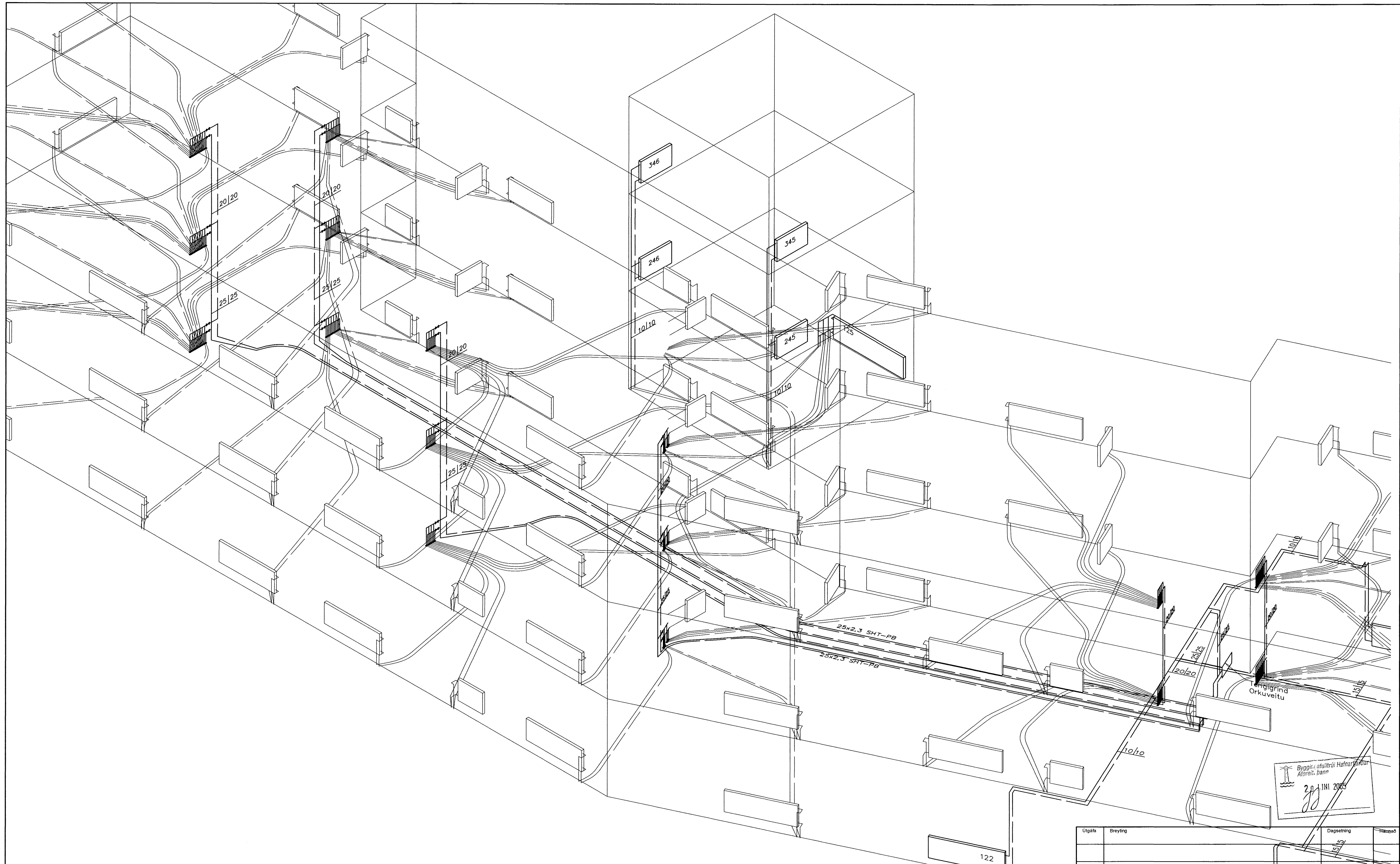
Hitalagnir, Rúmmynd, 1:50
