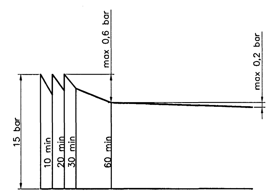
Þrýstiprófun á neysluvatnslögnum línurit
