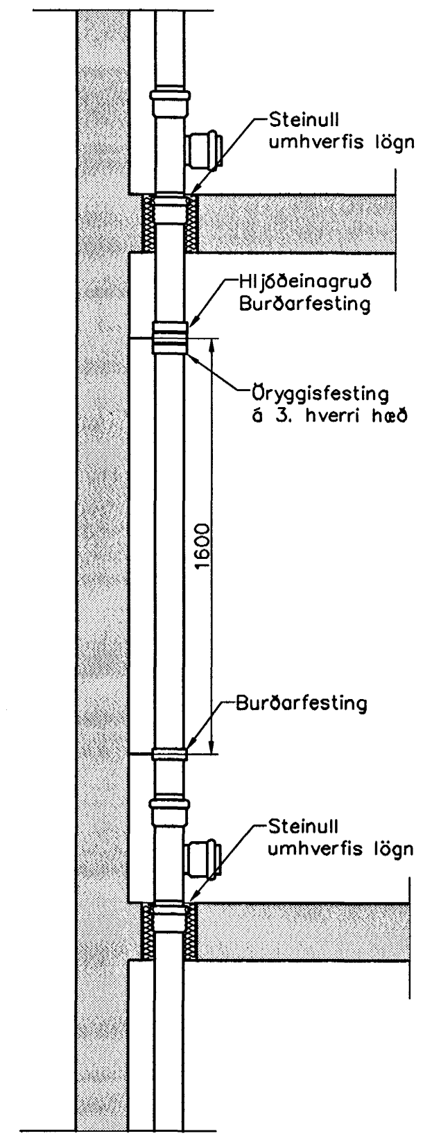
Fallpípa, festingar 1:20
