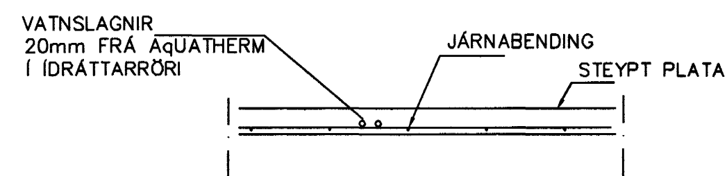
LAGNIR, SNIÐ, 1:20
