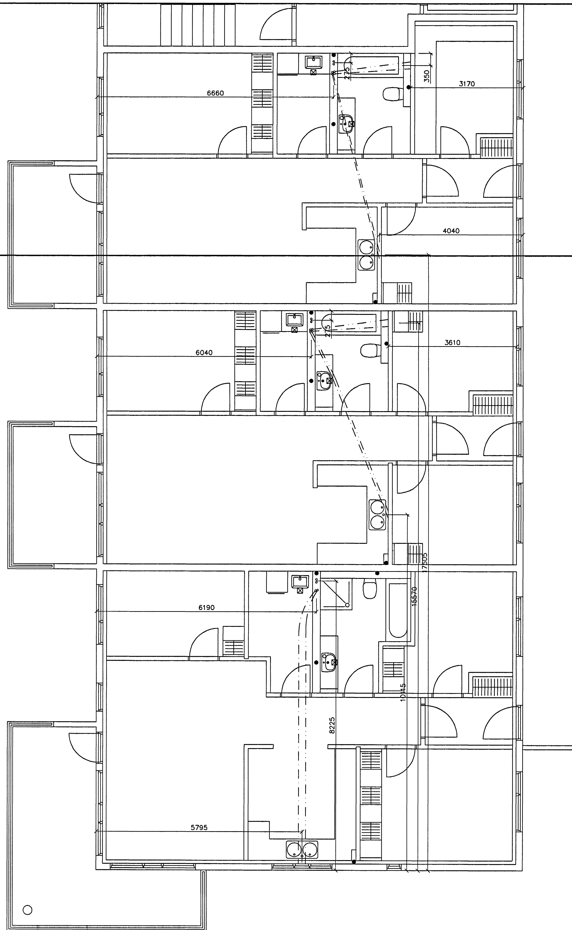
GRUNNMYND 4 HÆÐAR 1:50
