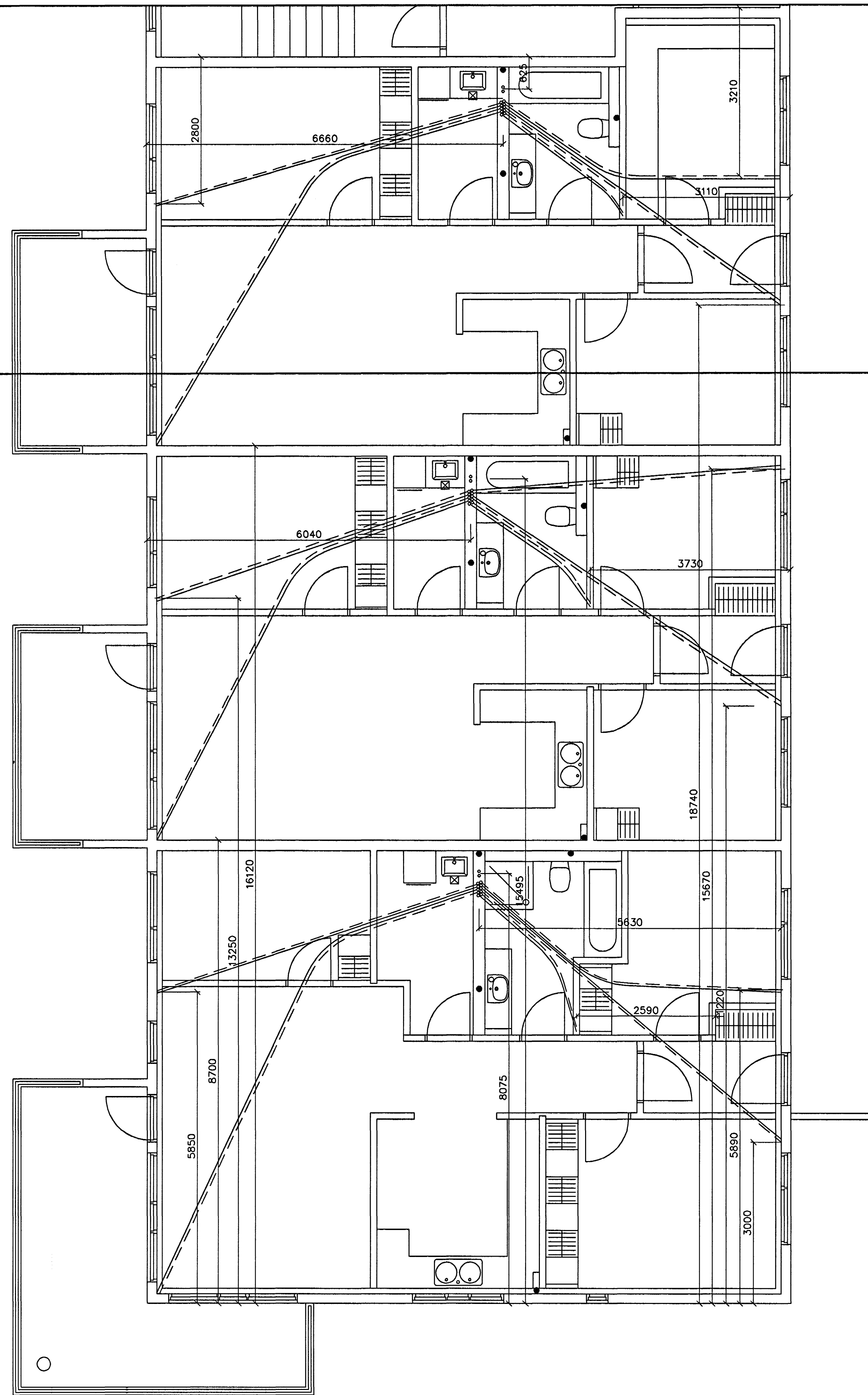
GRUNNMYND 4 HÆÐAR 1:50
