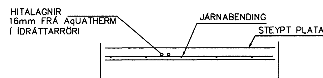
LAGNIR, SNIÐ, 1:20
