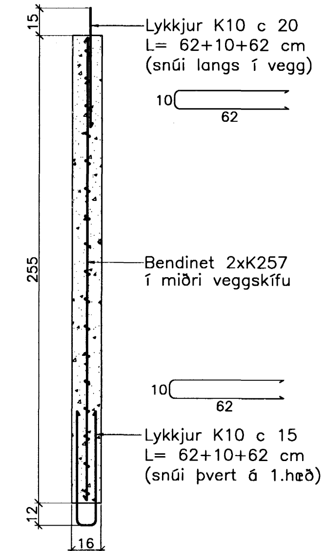
Snið W-W
