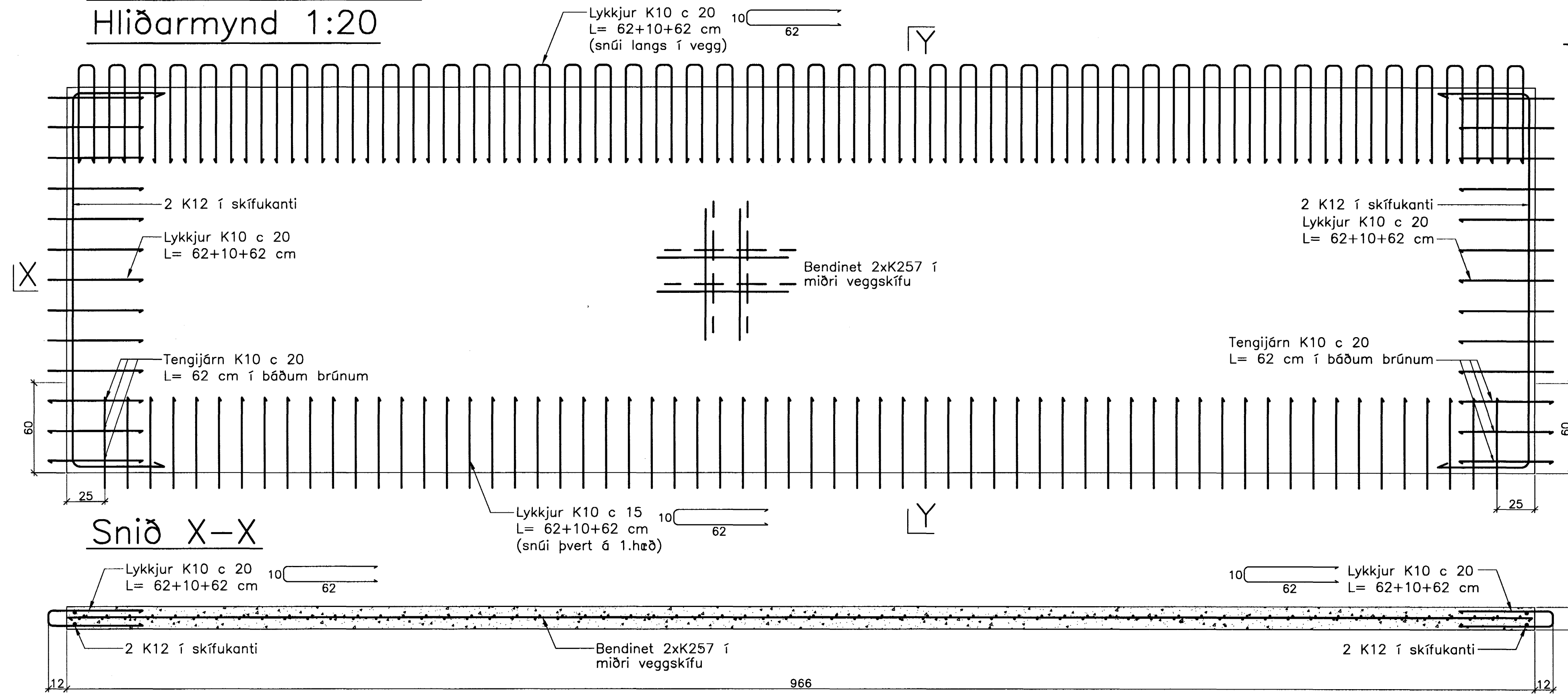
Innveggur IV.1.2.32 Hliðarmynd 1:20
