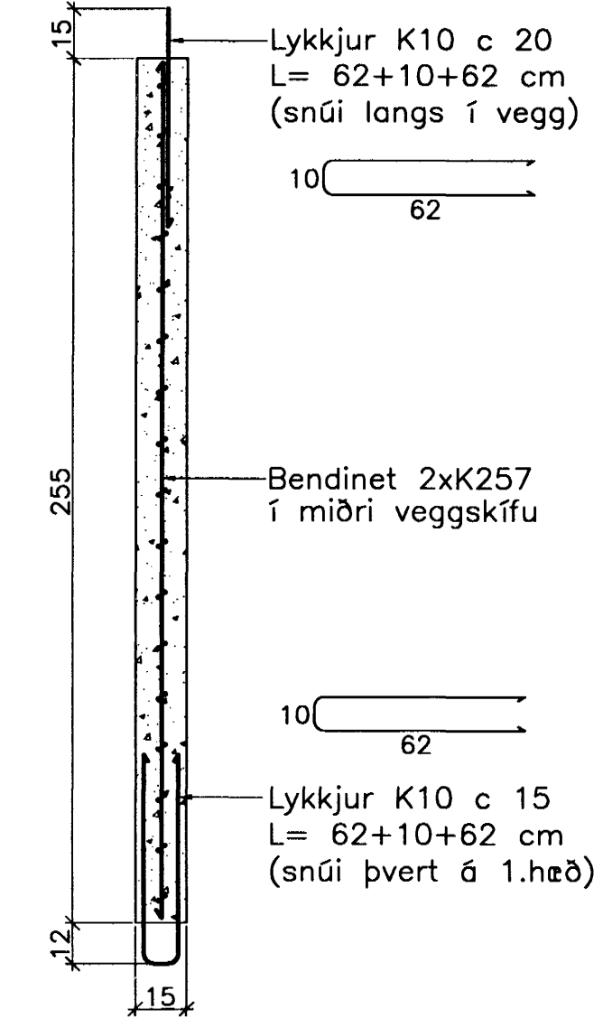
Snið Y-Y
