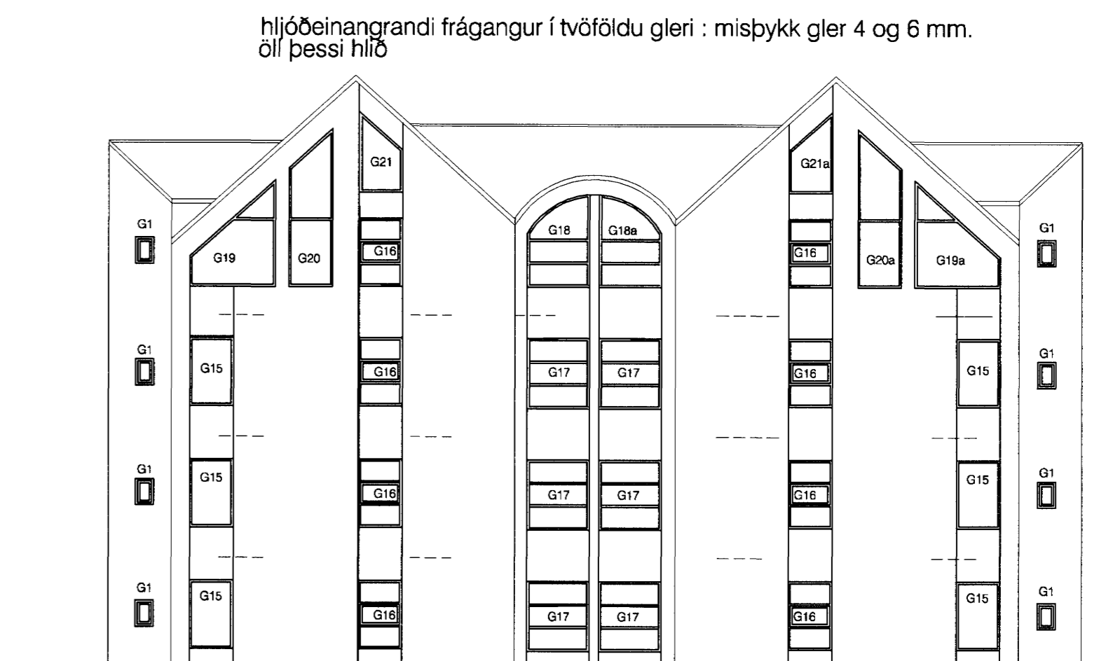
útlit norðaustur
