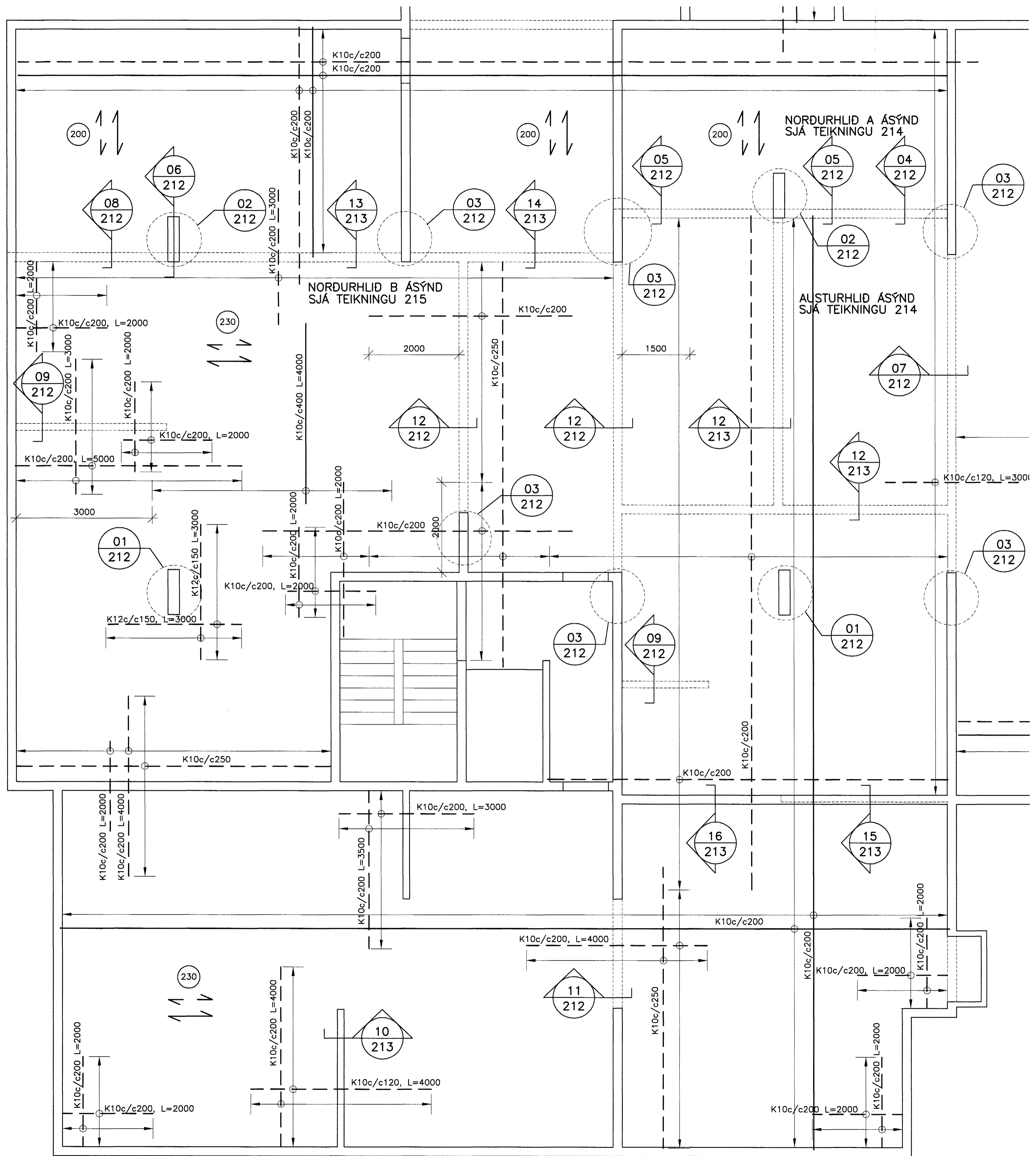
GRUNNMYND 1:50
