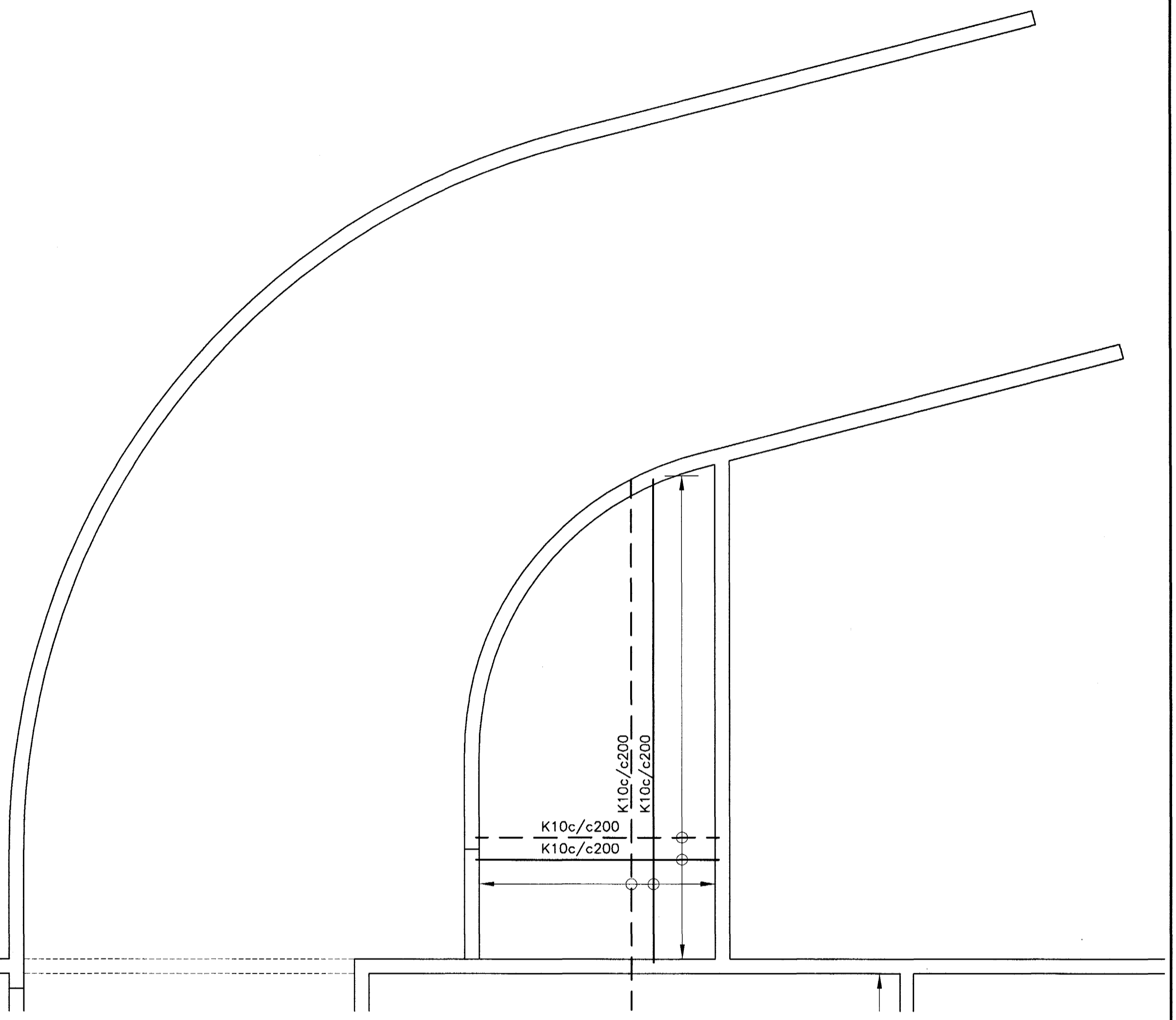
GRUNNMYND 1:50
