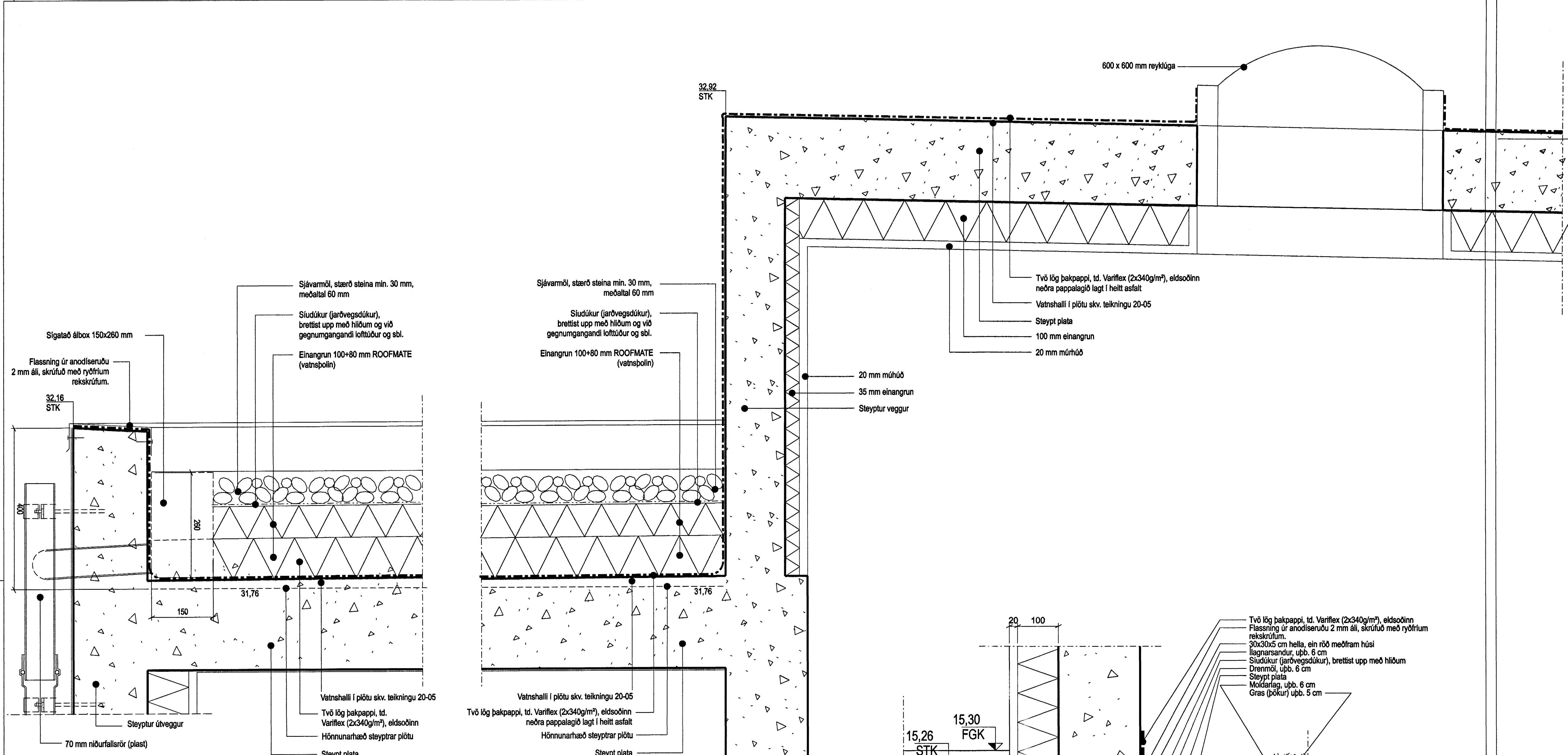
1 DEILI 1:5 20-20 Frágangur þaks við útvegg 20-21
