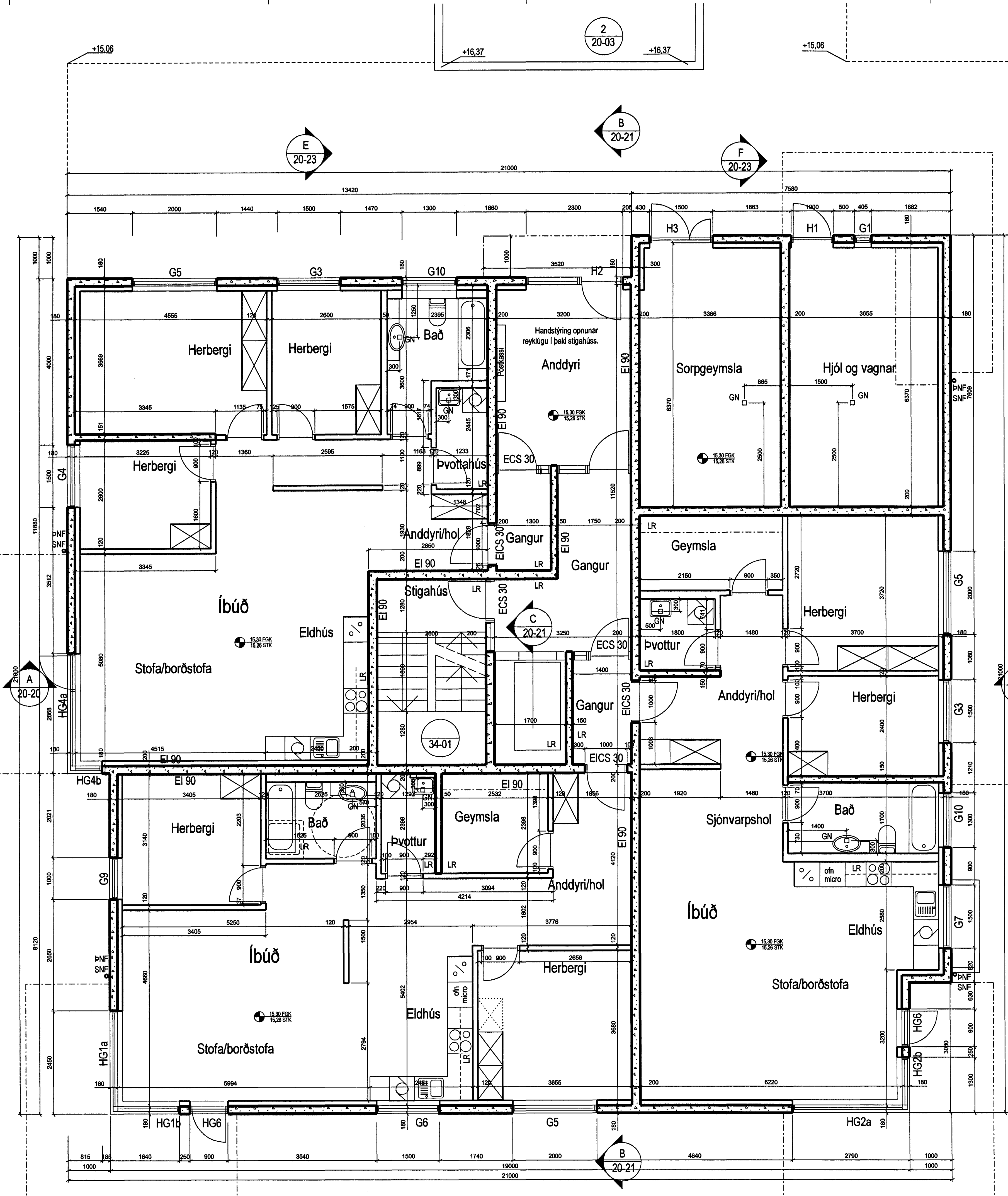
1 GRUNNMYND 1:50 Grunnmynd 1. hæð
