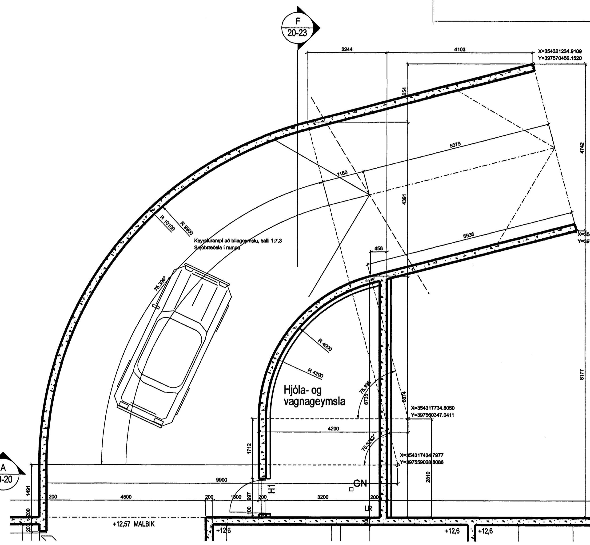
2 GRUNNMYND 1:50 Grunnmynd rampa og sorggeymslu
