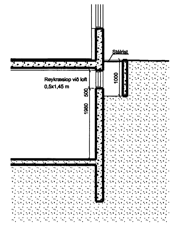
3 SNEIÐING 1:50 Hlutansneiðing í vegg við reykraup
