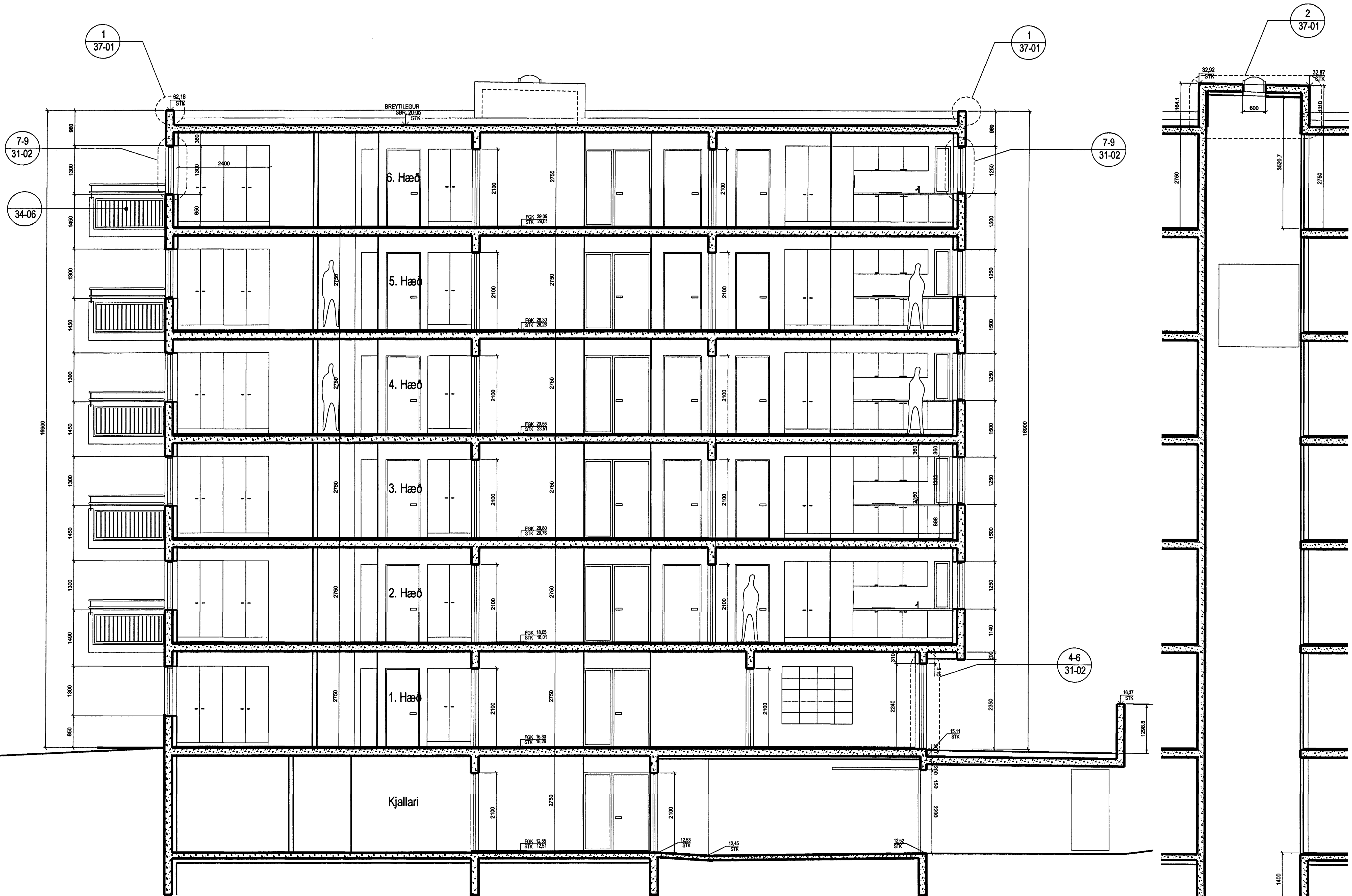
B-B 20-01 SNEIDING 1:50 20-02, 20-03, 20-04
