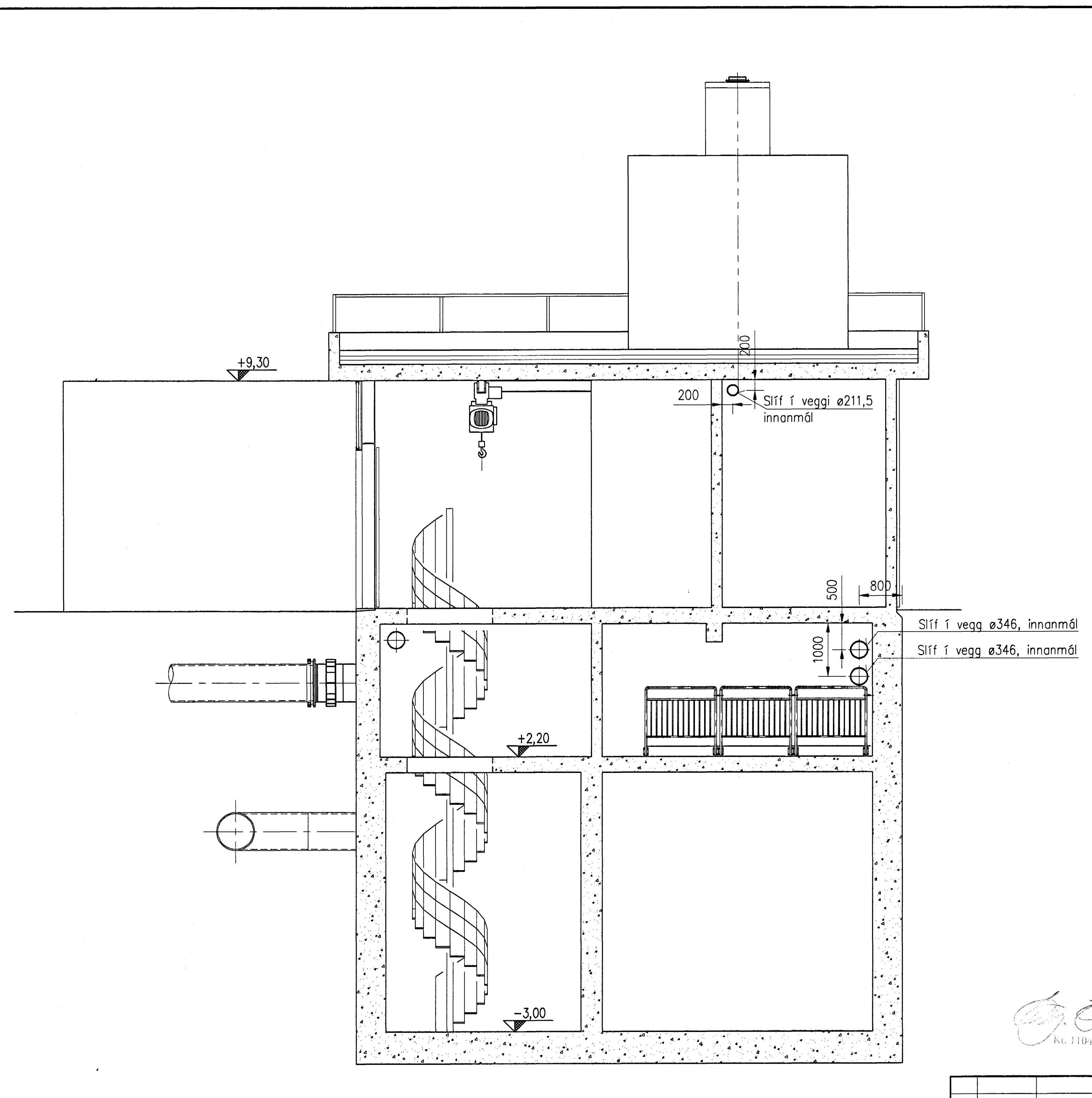
D SNÍÐ D-D
