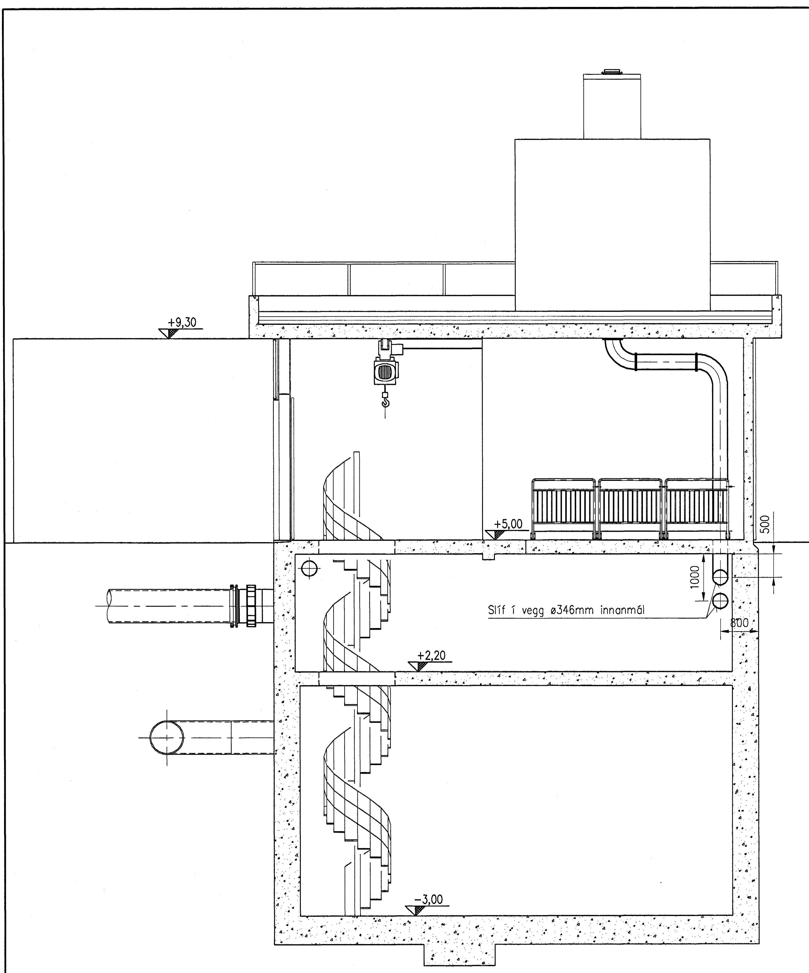
C SNÍÐ C-C
