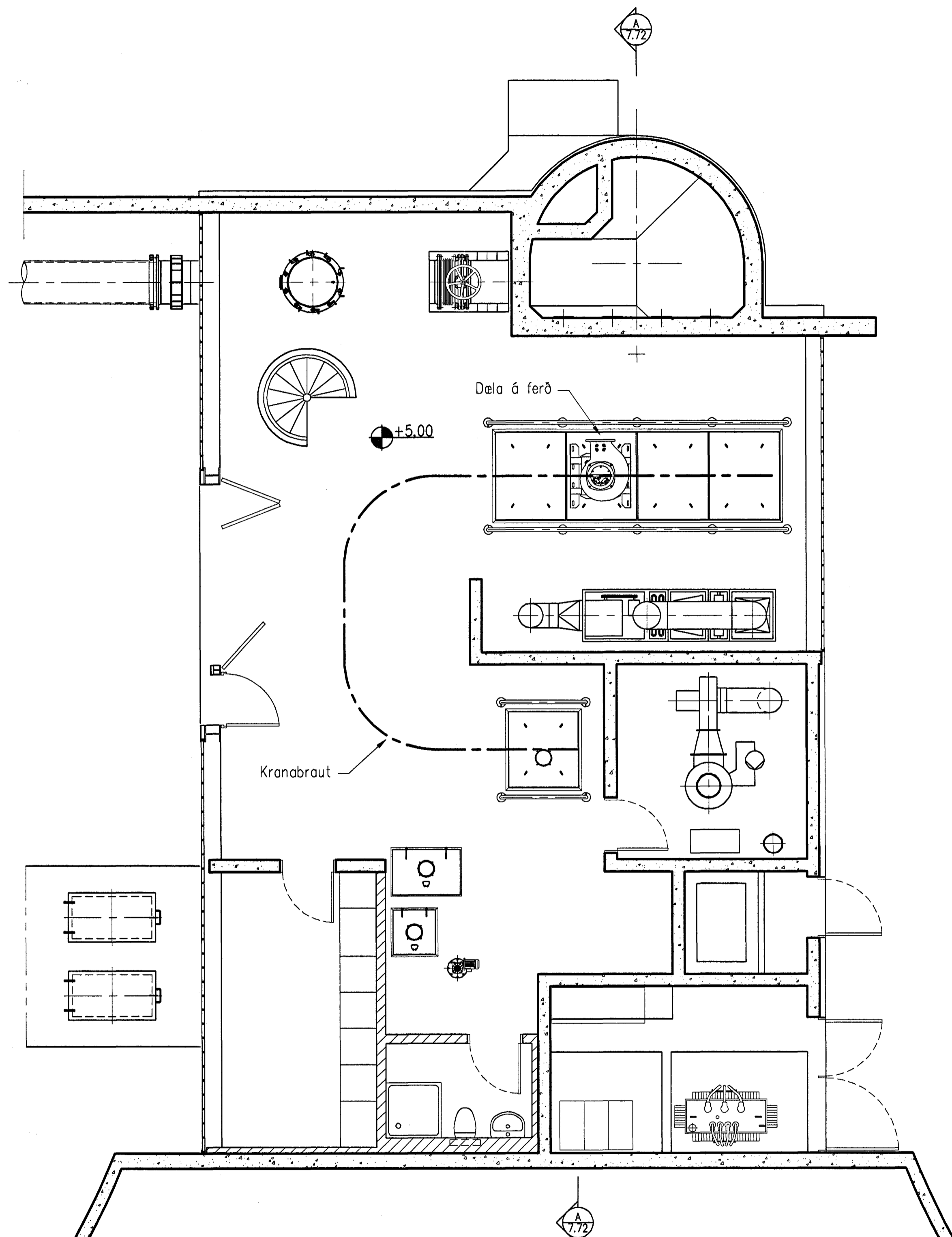
GRUNNMYND EFRA RÝMIS
