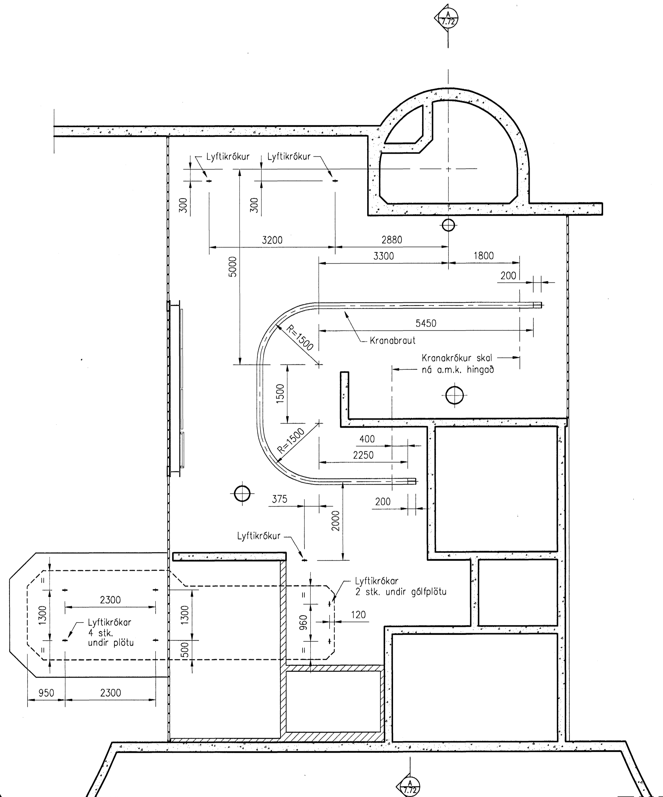
SNIÐ Í EFRA RÝMI VIÐ LOFT
