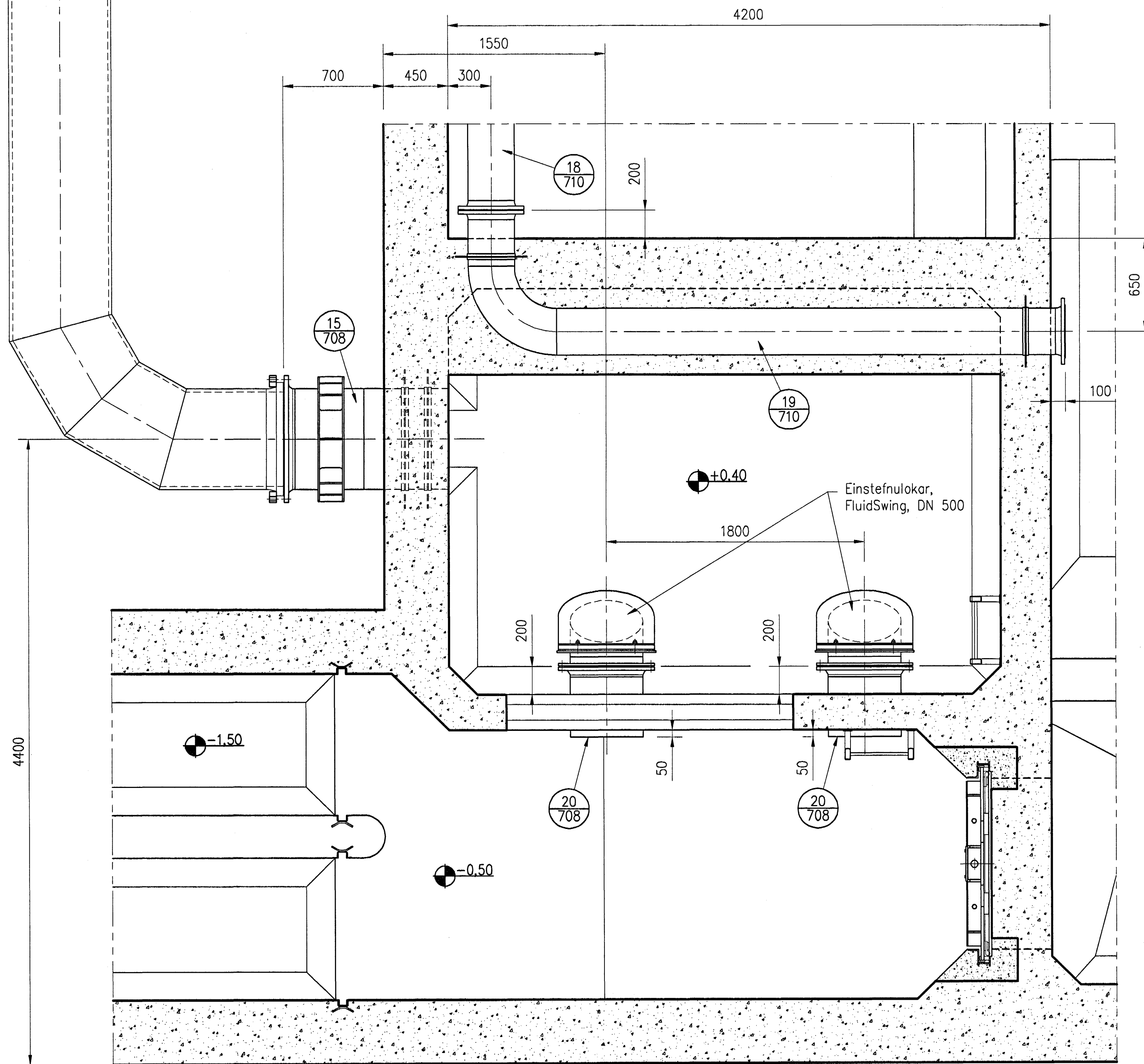
— — LÁRÉTT SNIÐ
