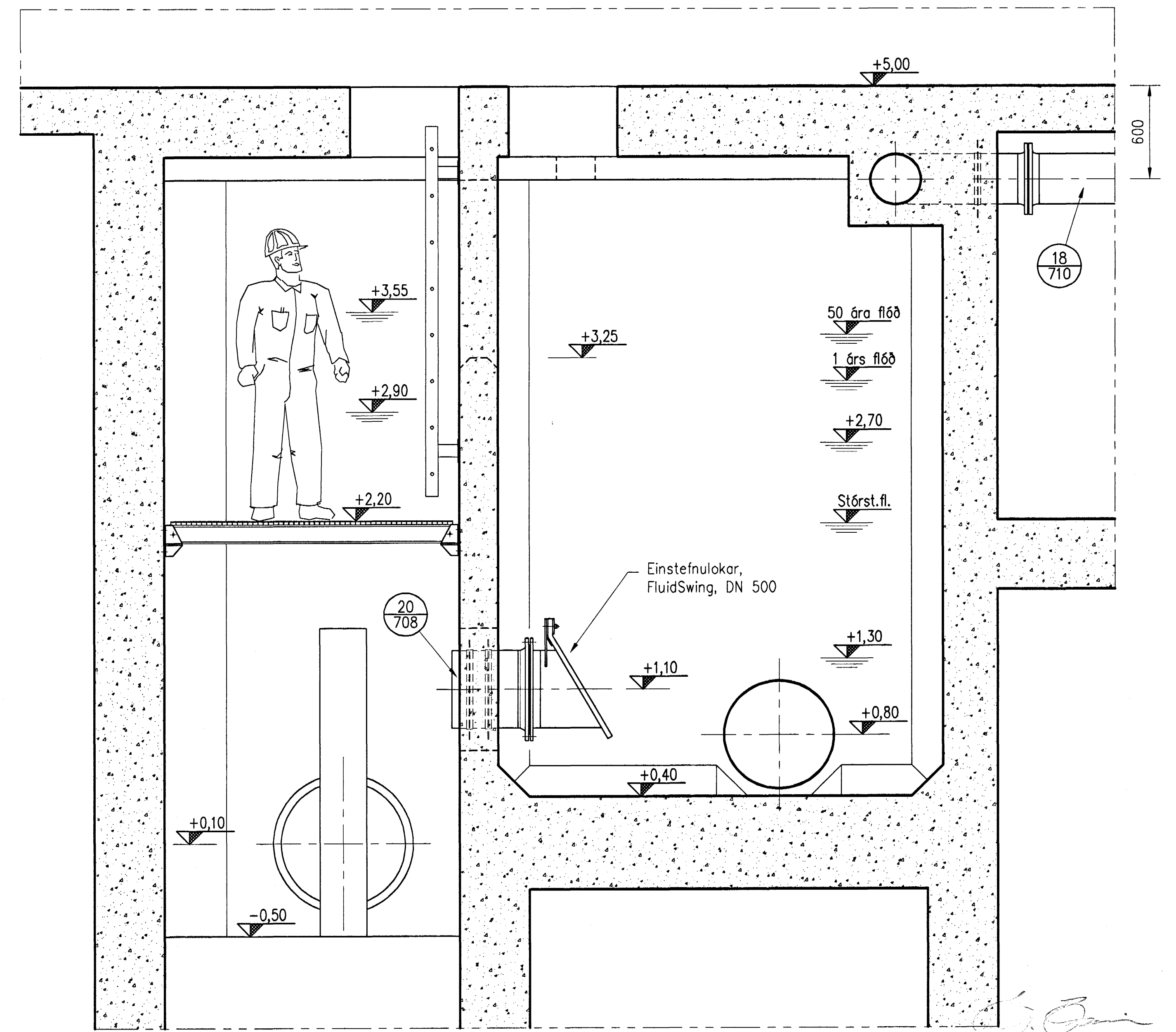
— — LÖDRÉTT SNIÐ
