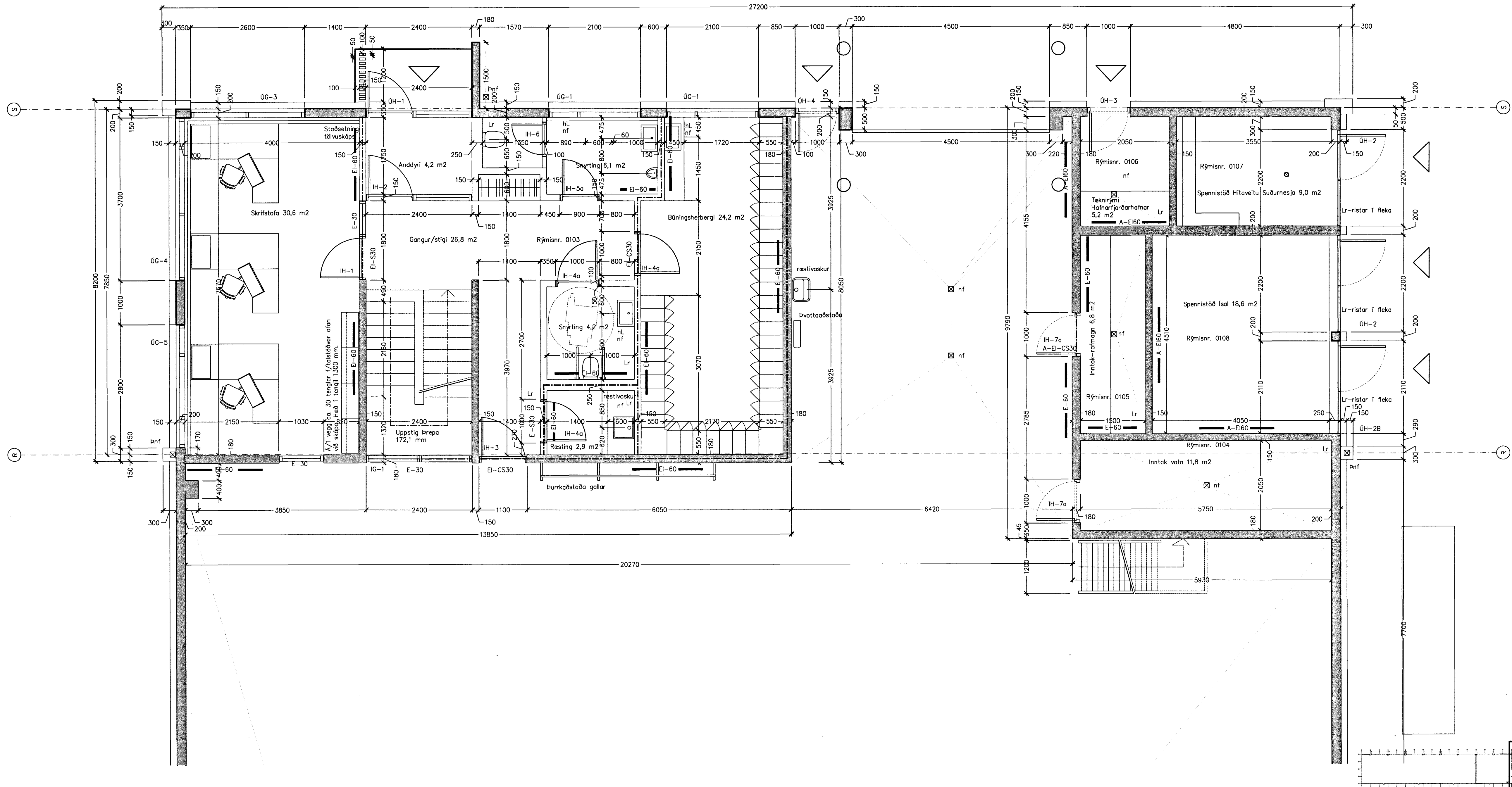
Grunnmynd starfsmannarými 1. hæðar mkv. 1: 50
