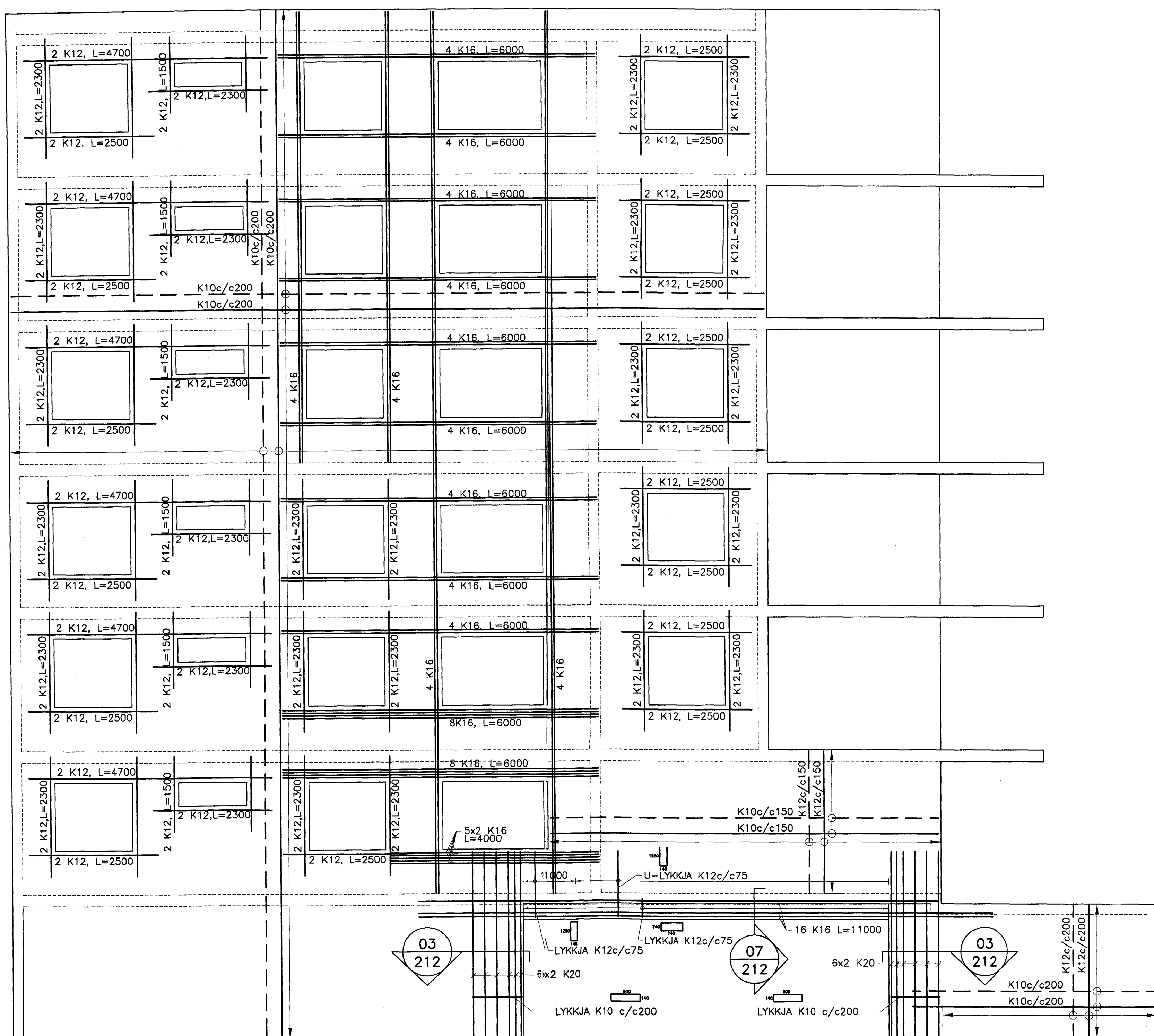
ASÝND AUSTURHLID 1:50
