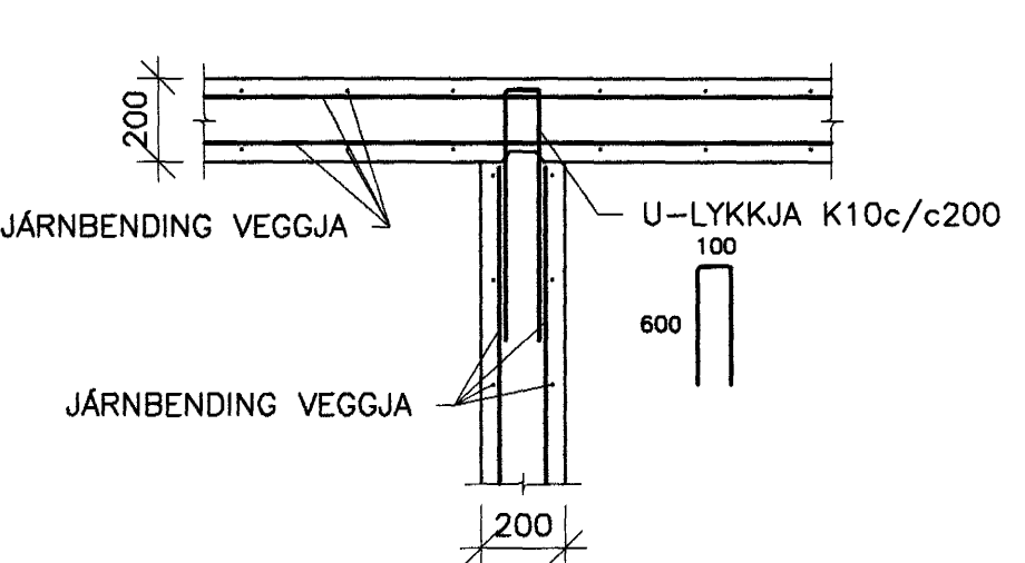
TENING VEGGJA. 1:20
