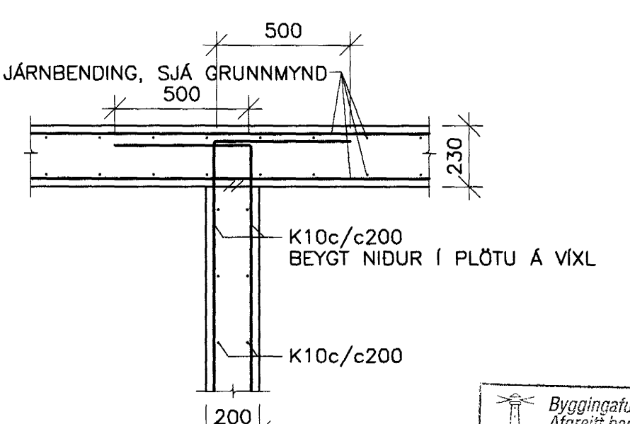
16 SNID 211 212 1:20
