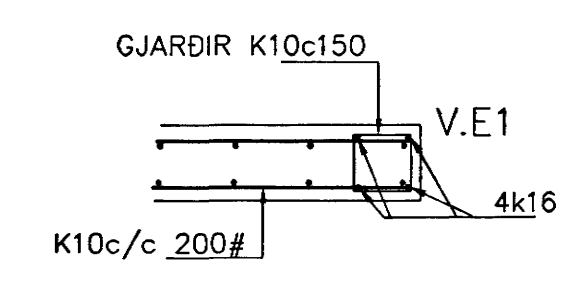
VEGGENDAR 1:20
