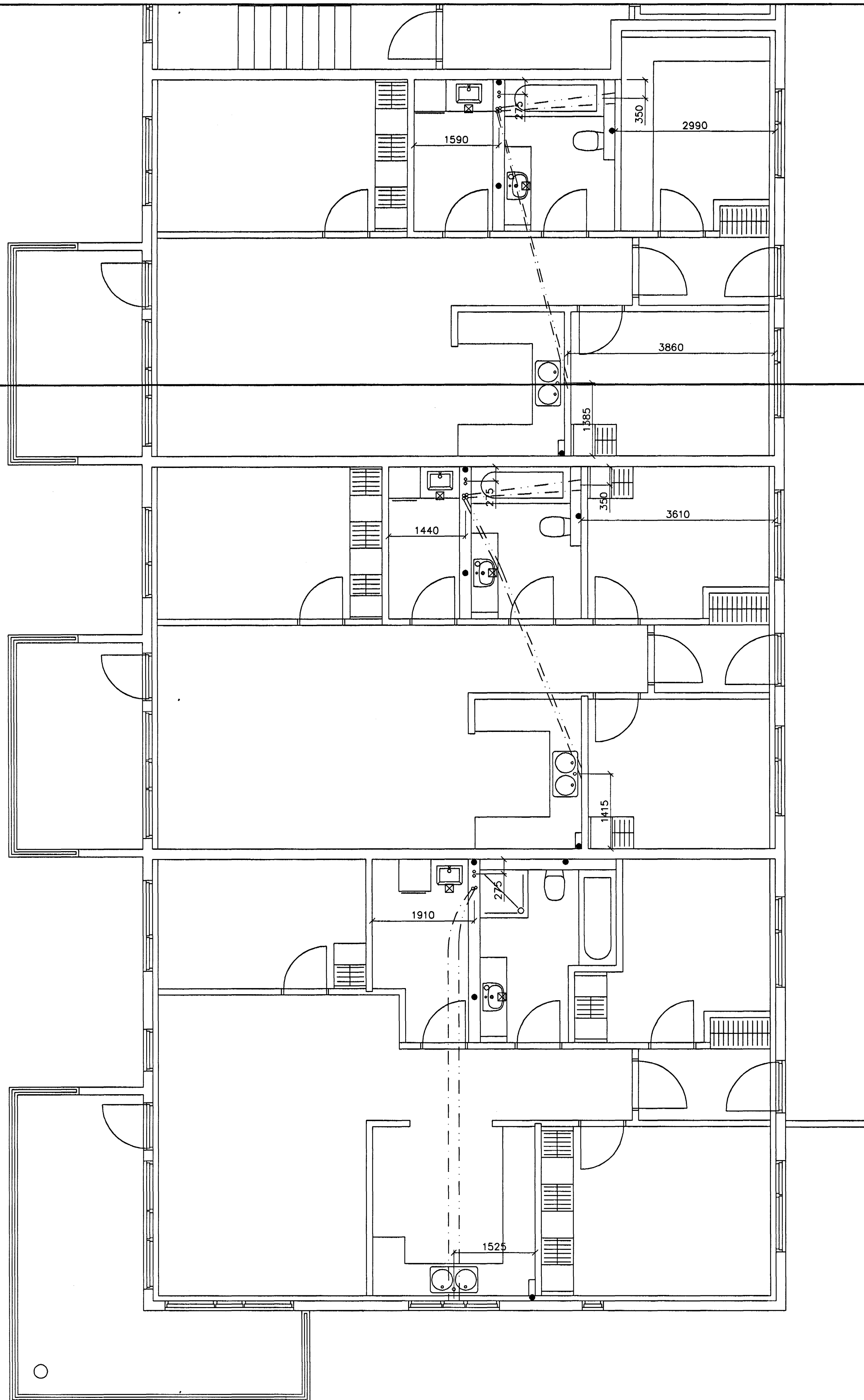
GRUNNMYND 2 HÆÐAR 1:50
