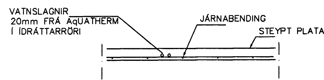
LAGNIR, SNIÐ, 1:20
