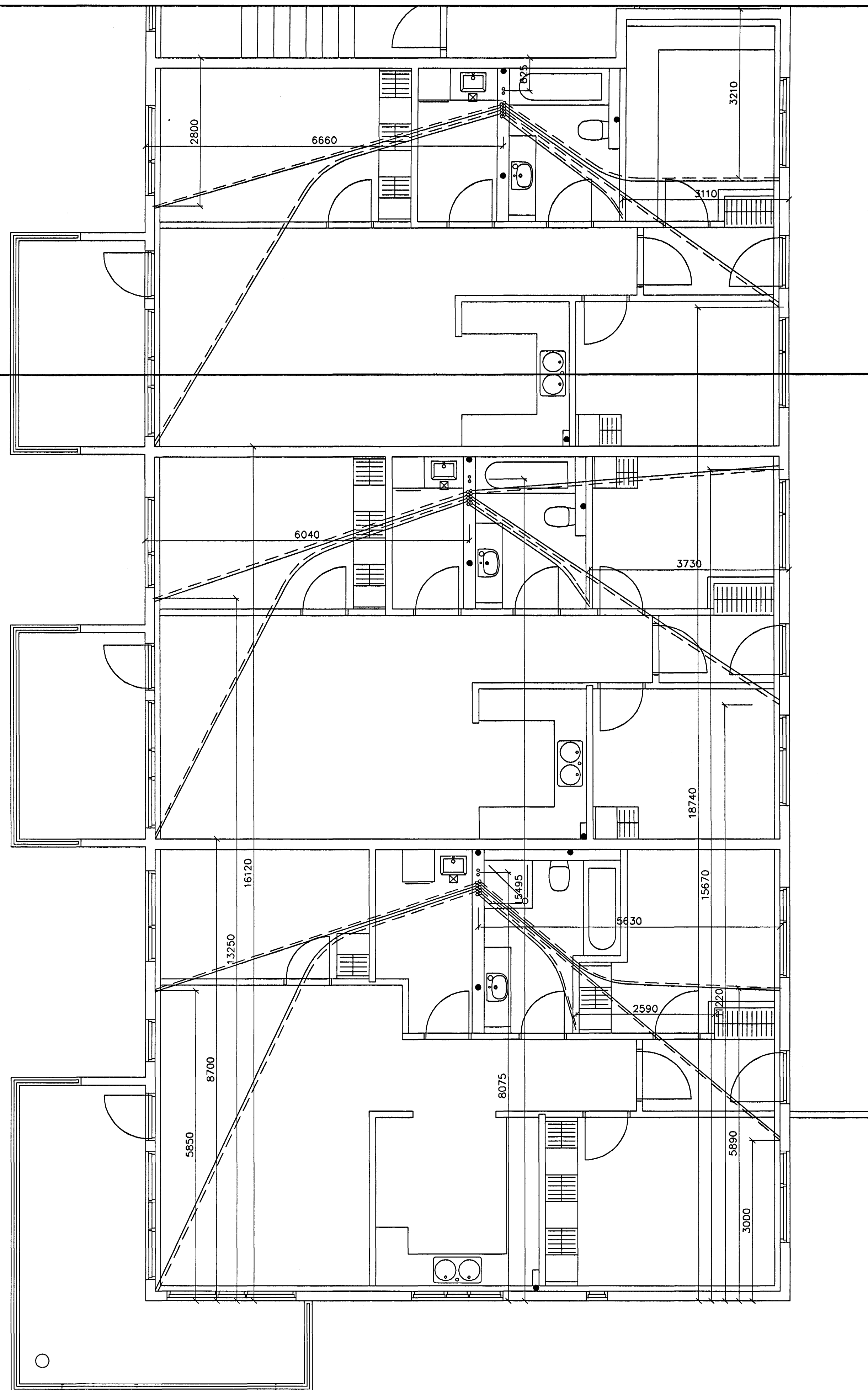
GRUNNMYND 2 HÆÐAR 1:50
