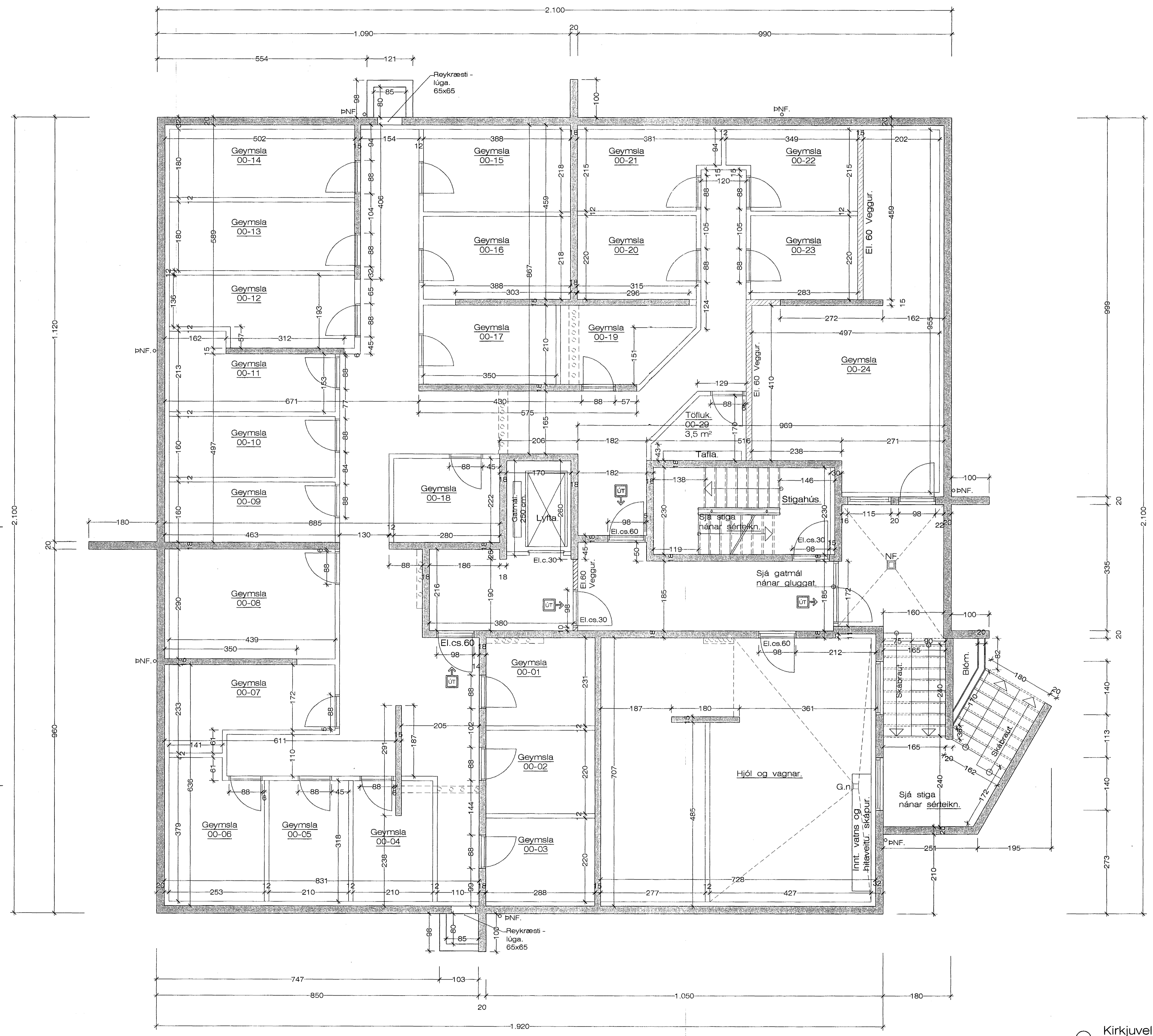
Grunnmynd kjallara. 1:50
