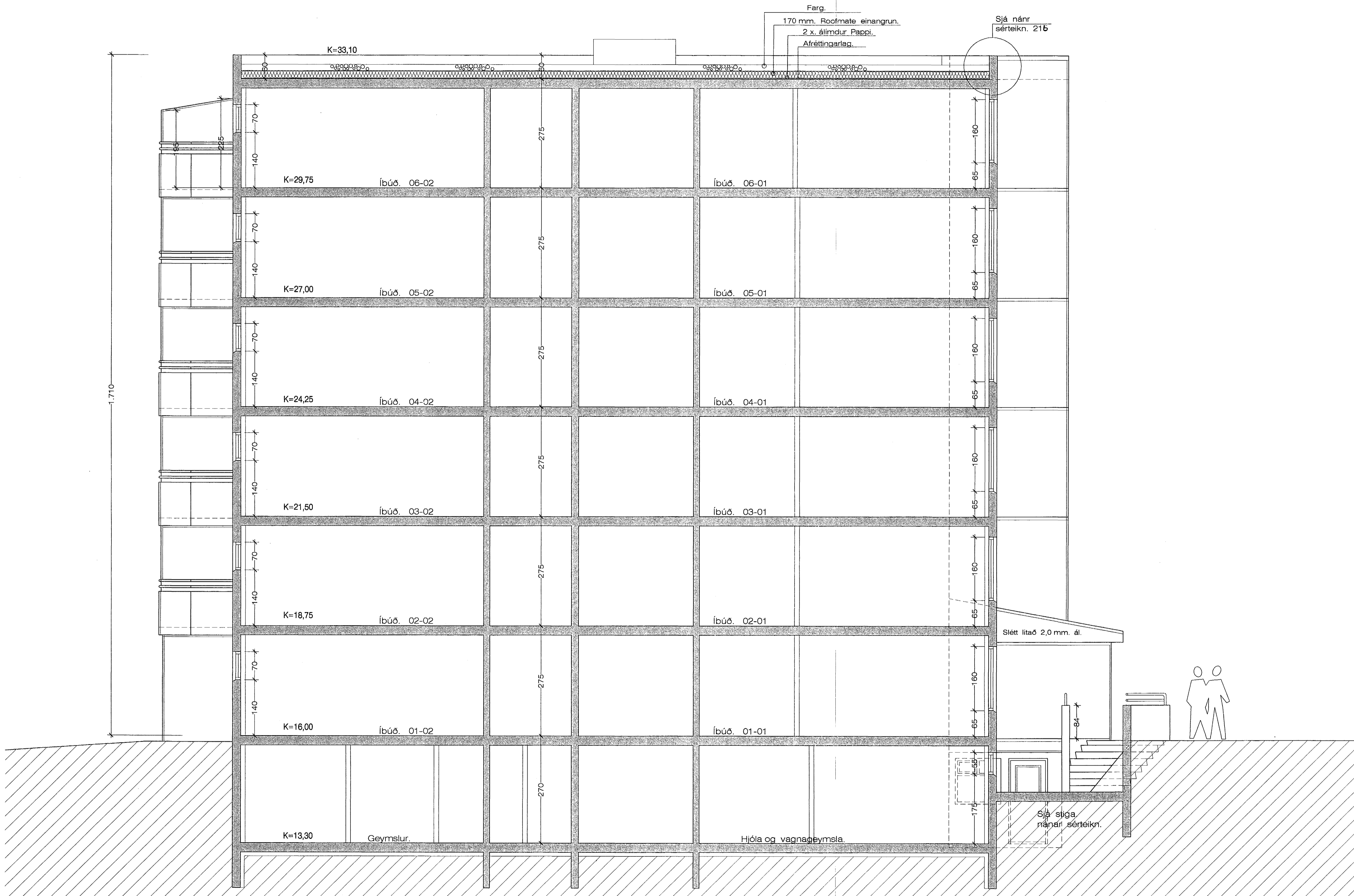
Sneiðing. A - A 1:50
