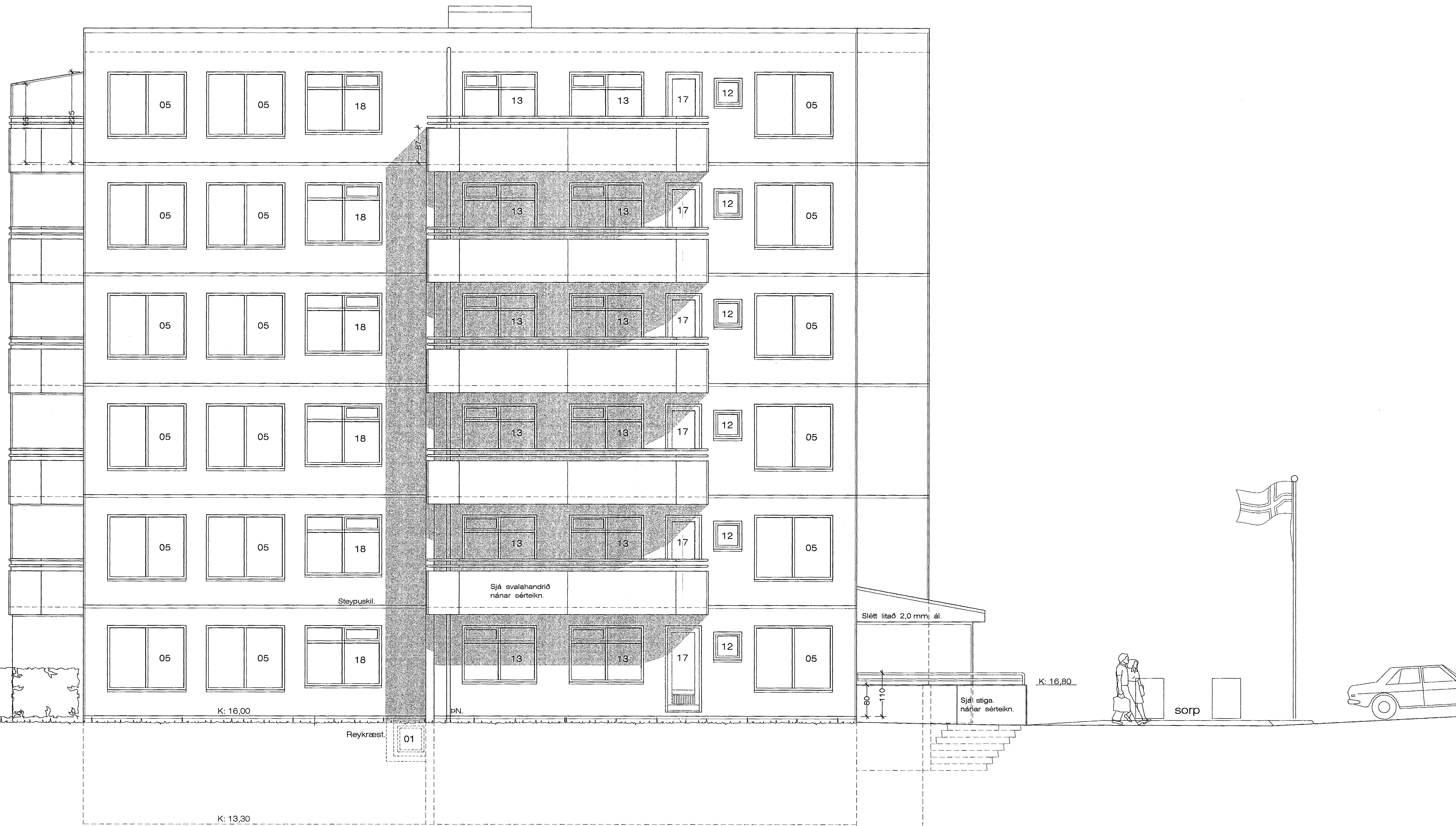
Suðurhlið. 1:50
