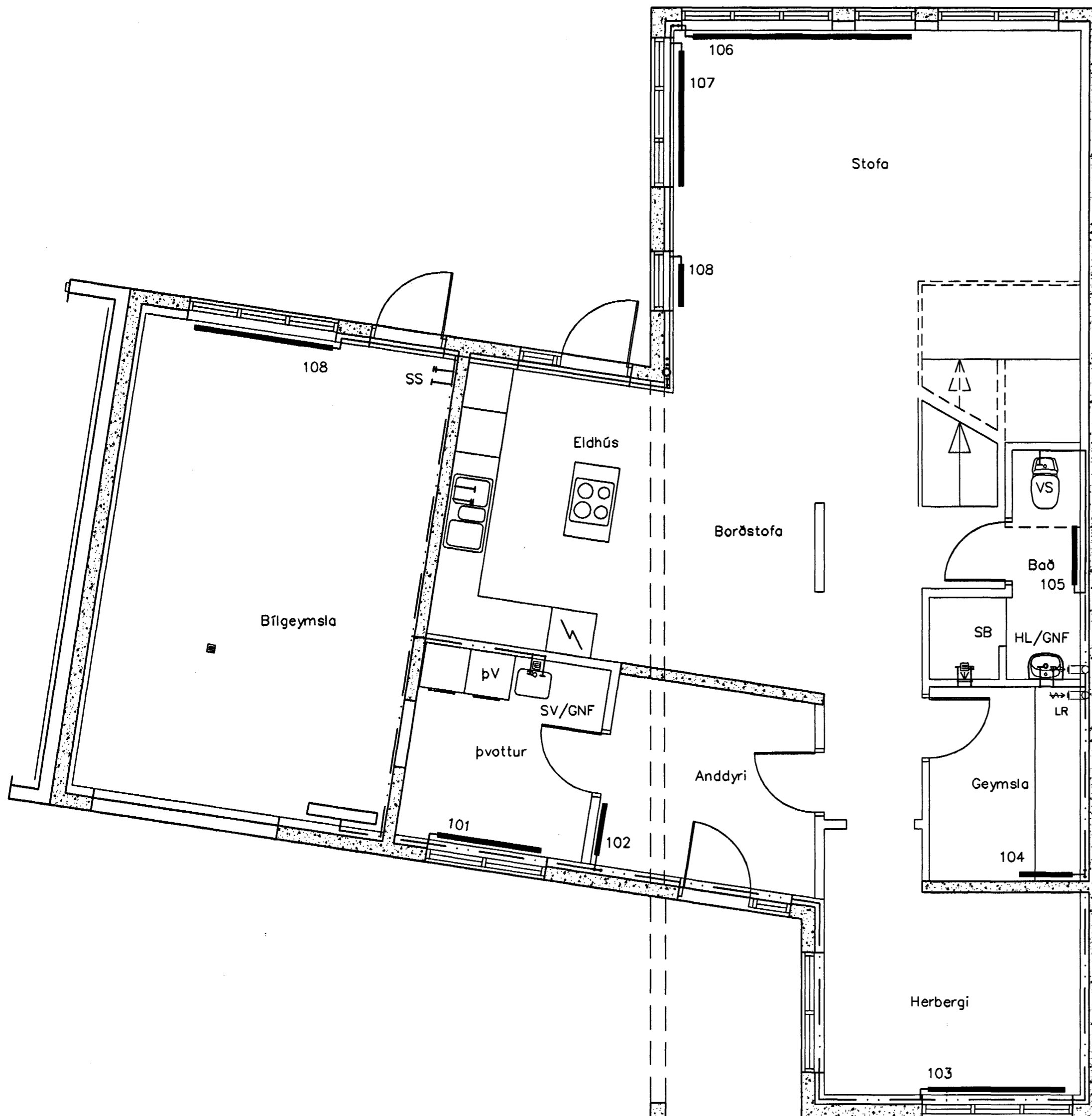
Lagnir 1. hæð, 1:50
