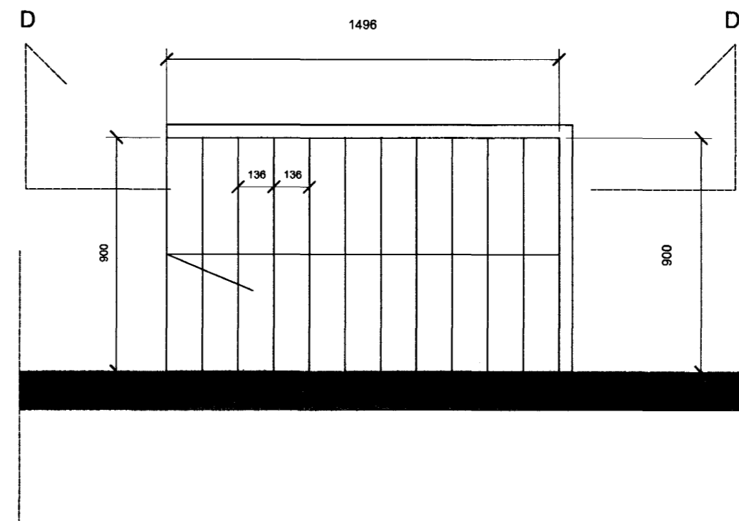
Grunnmynd stigi
