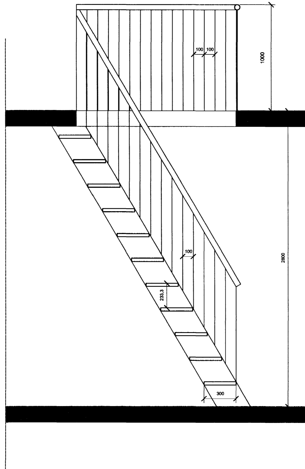
Sneiðing í stiga D-D
