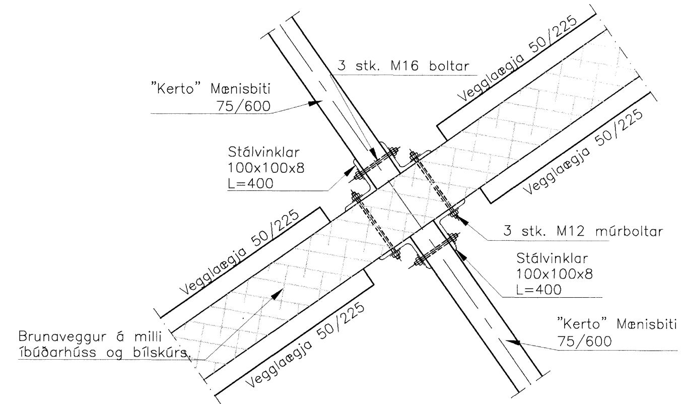
C FESTING BITA VID VEGG 201202 M. 1:10
