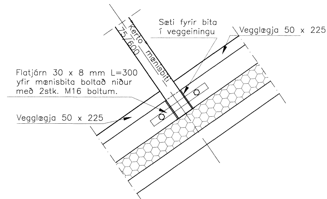
D FESTING MÆNISBITA 201202 M. 1:10
