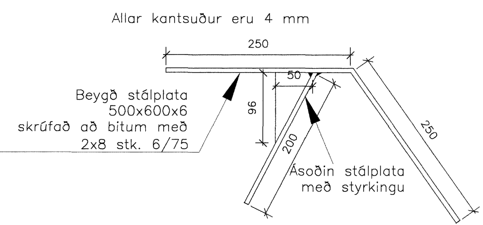
Sérmynd 1 Stáiplata mkv. 1:5
