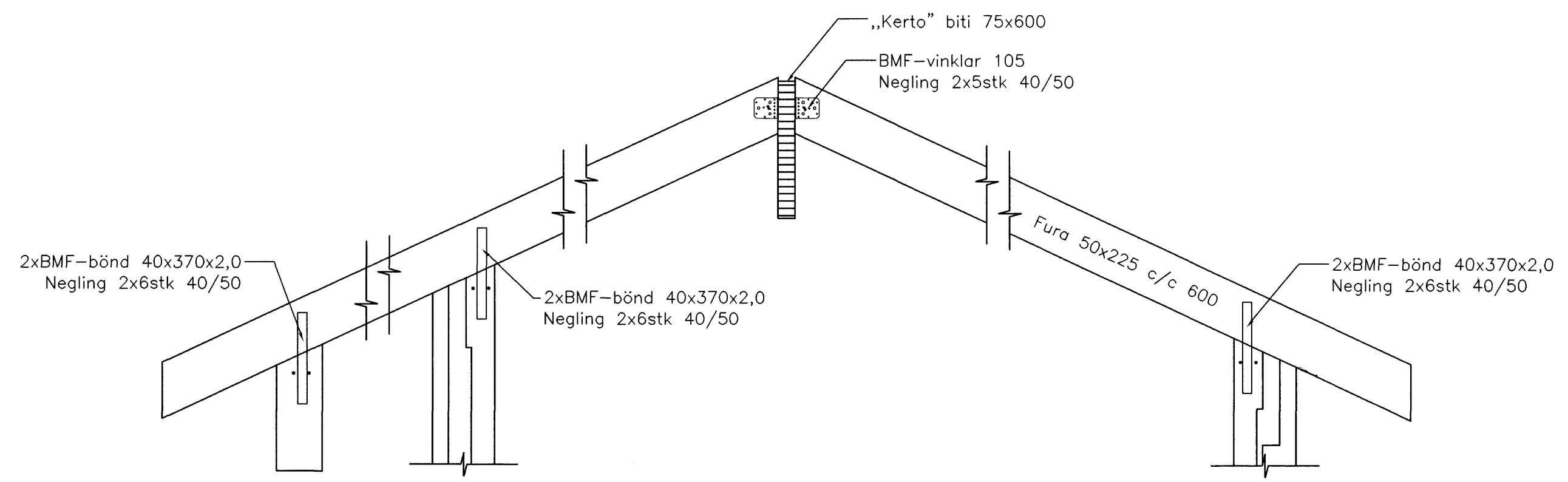
2 SNID 201202 M. 1:20
