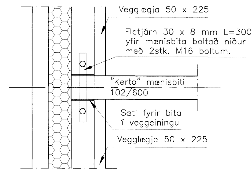
A FESTING MÆNISBITA 201202 M. 1:10
