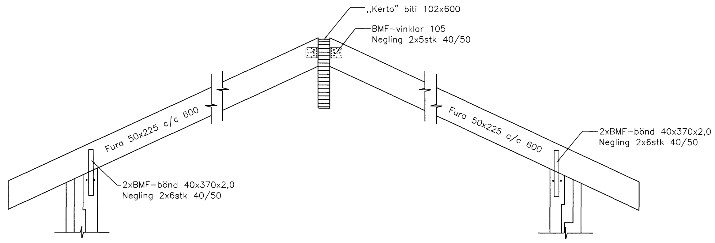
1 SNID 201202 M. 1:20
