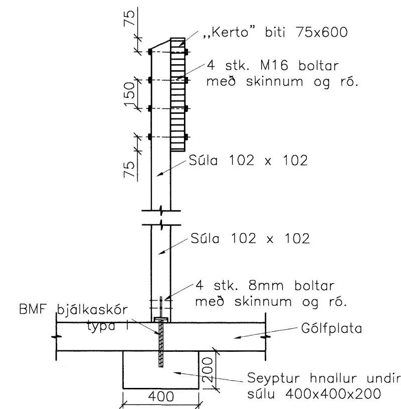
3 SNID 201202 M. 1:20
