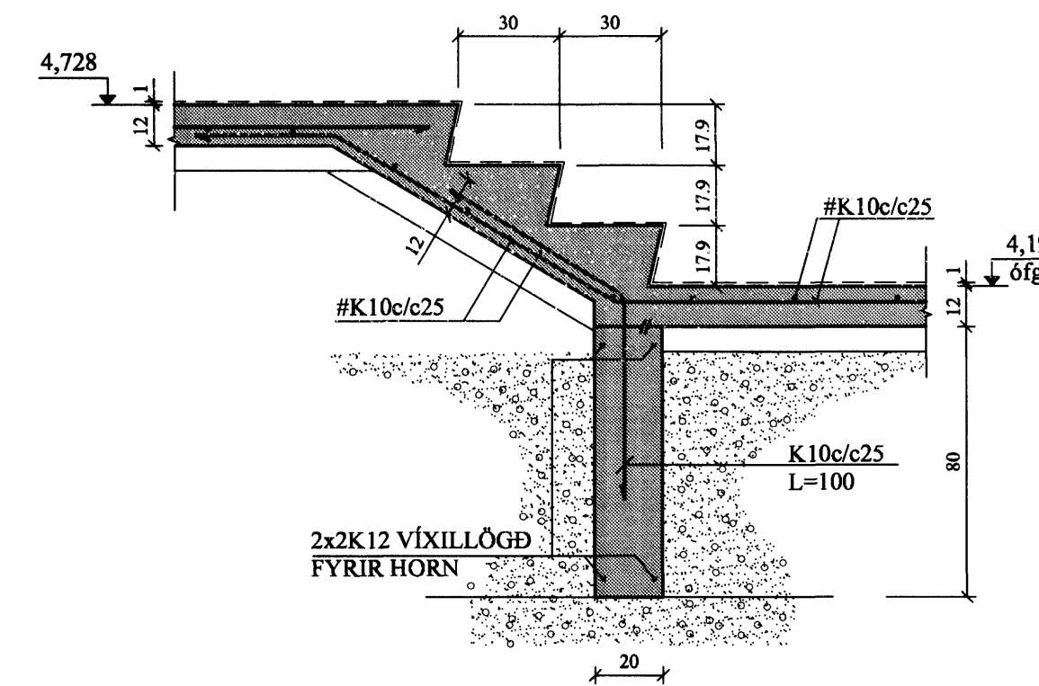
C2 SNIÐ. 1:20
