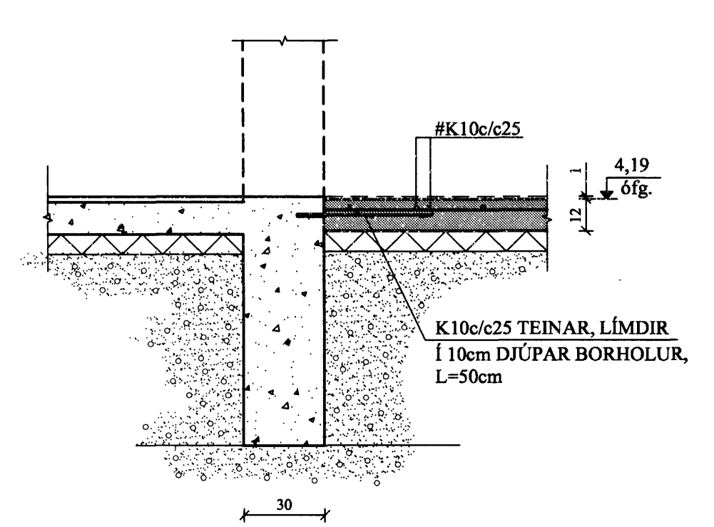
D2 SNIÐ. 1:20
