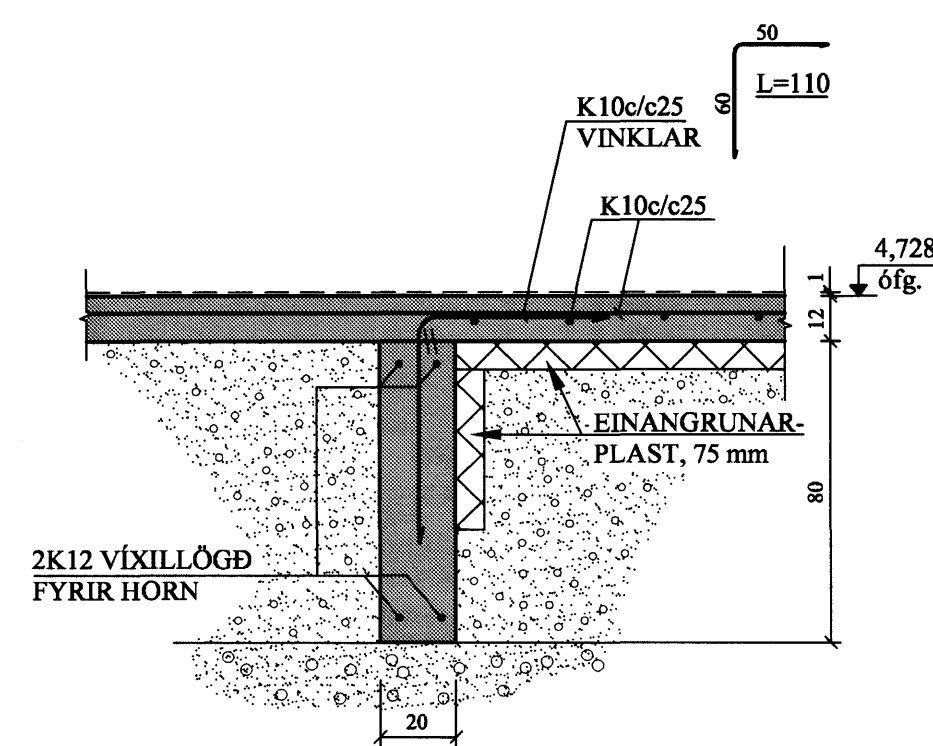
E2 SNIÐ. 1:20
