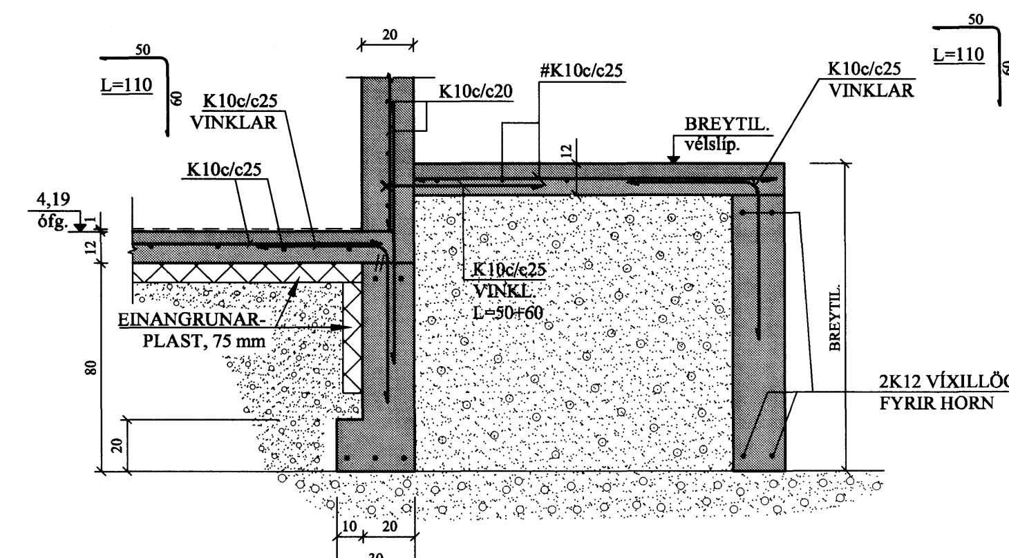
F2 SNIÐ. 1:20
