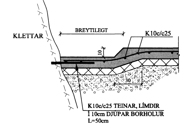
B2 SNIÐ. 1:20
