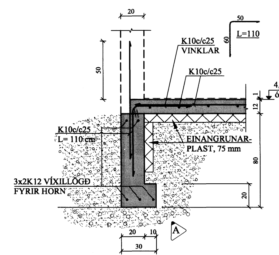
A2 SNIÐ. 1:20
