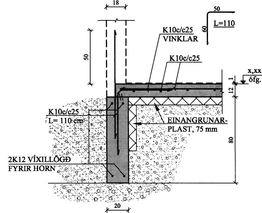
F2 SNIÐ. 1:20
