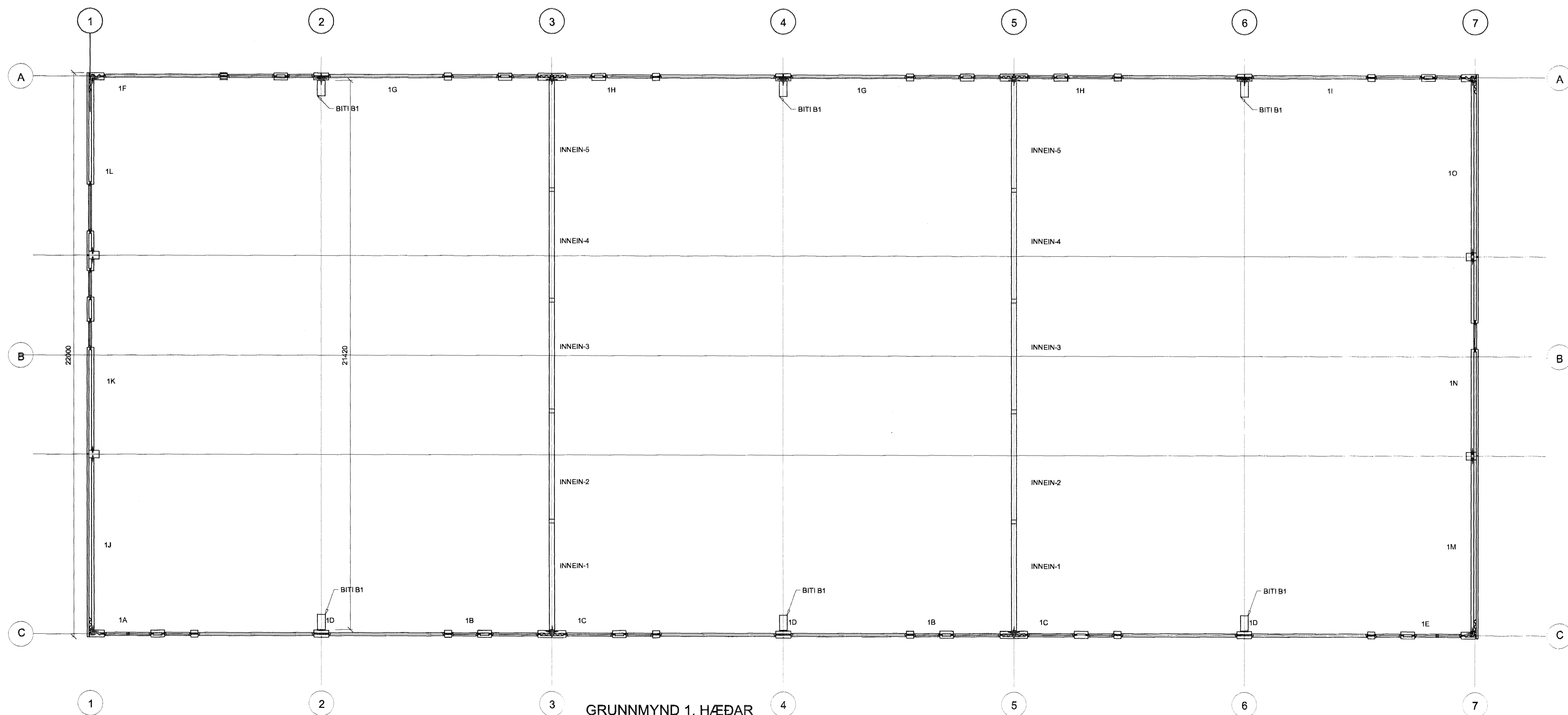
GRUNNMYND 1. HÆÐAR
