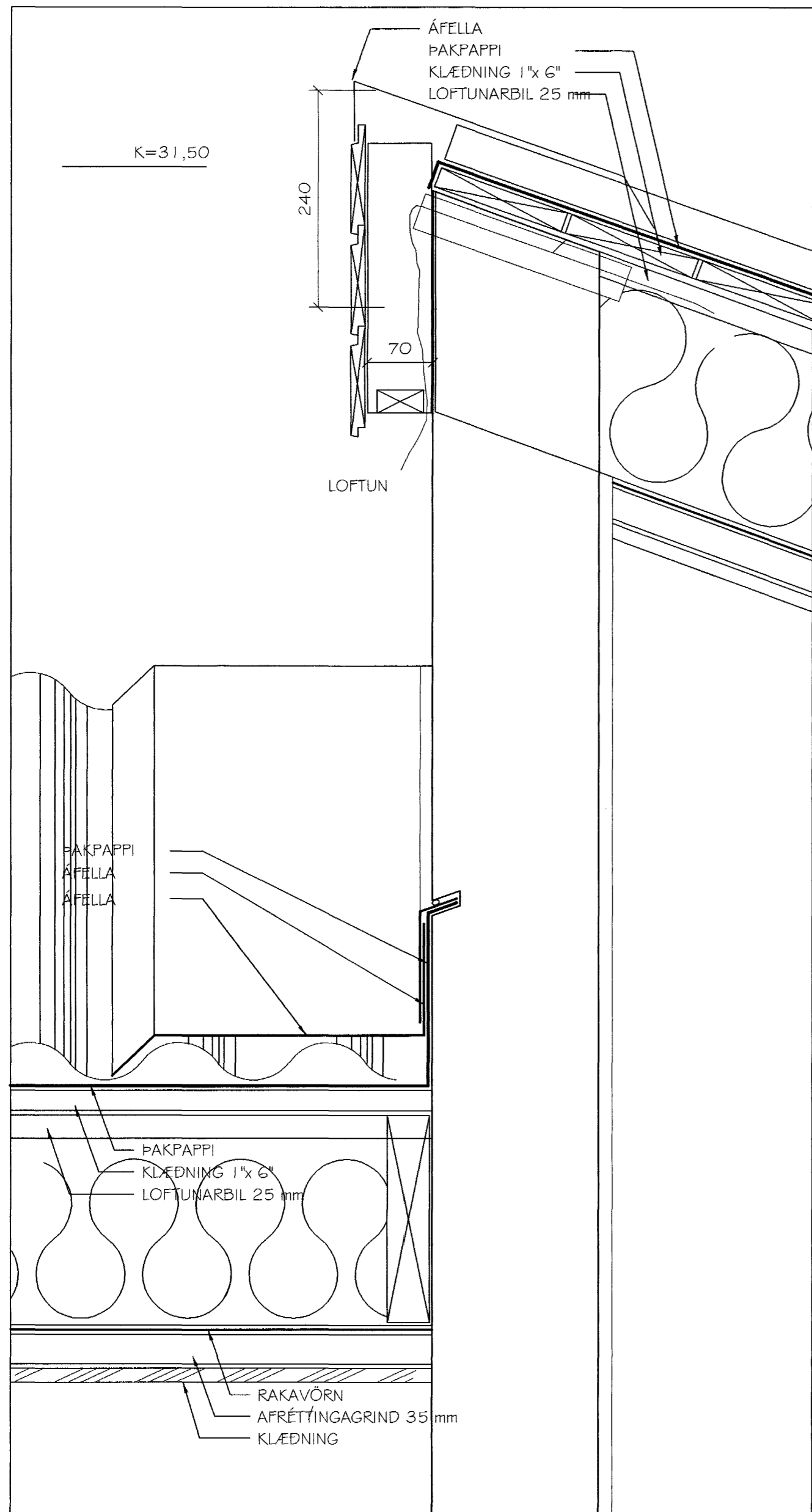
LÓDRÉTTISNEIÐING Í ÞAKFRÁGANG 1/5
