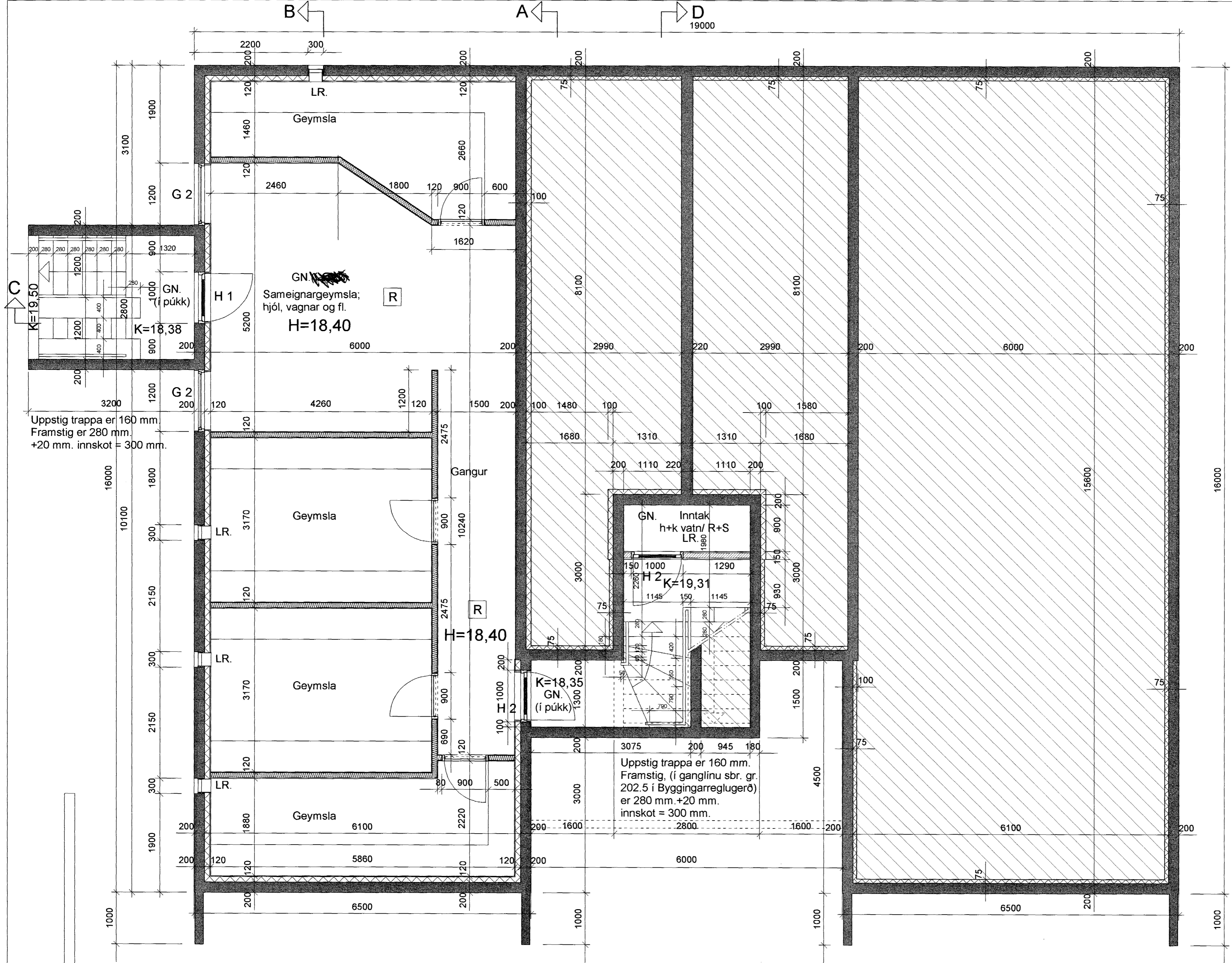
B ← A ← D → Grunnmynd kjallara
