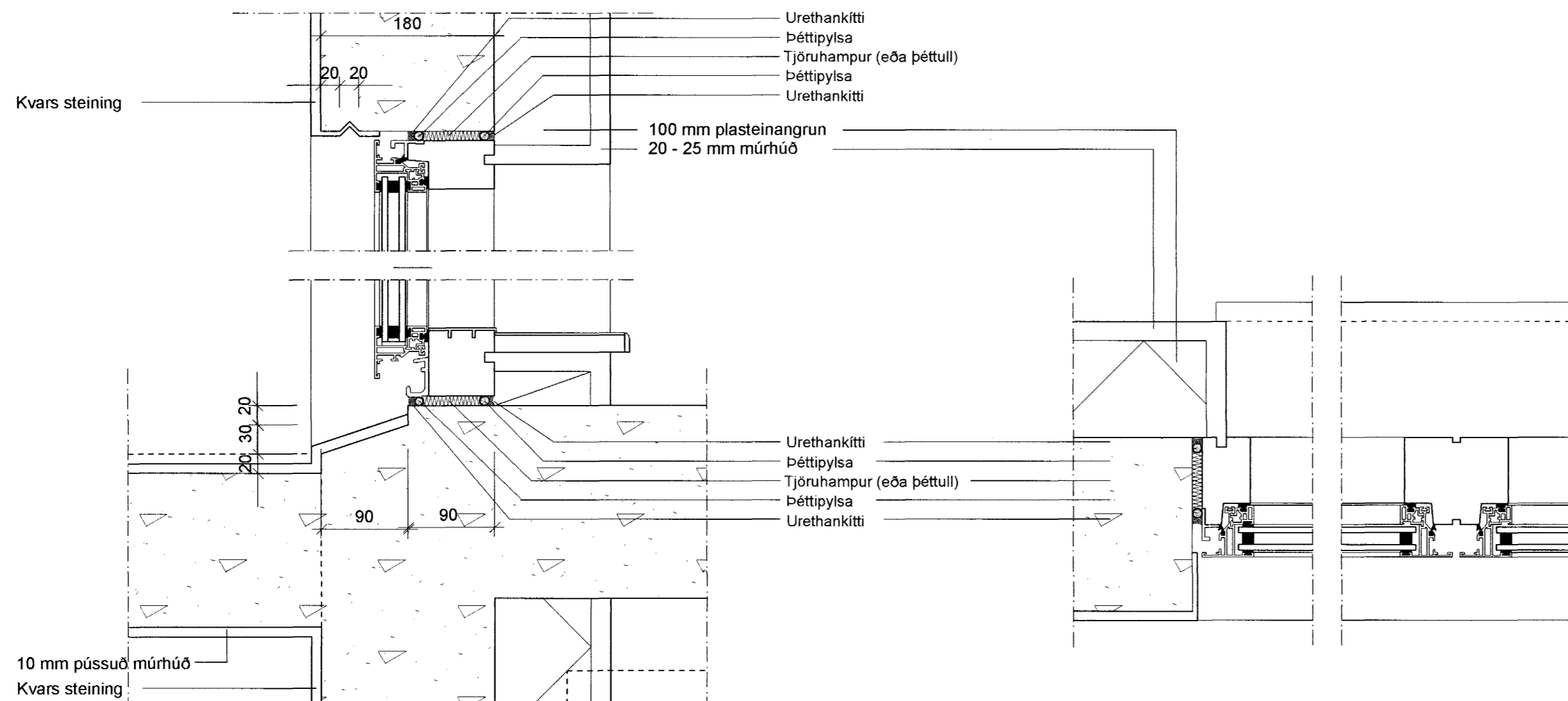
Frágangurdeili við HP 1, lóðréttur skurður 1:5
