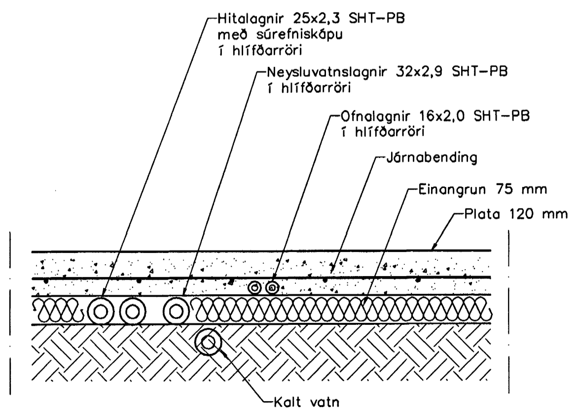
Hita- og Neysluvatnslagnir, Snið í botnplötu, 1:10
