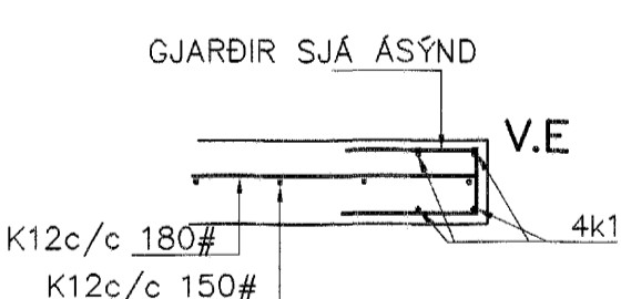
VEGGENDAR 1:20
