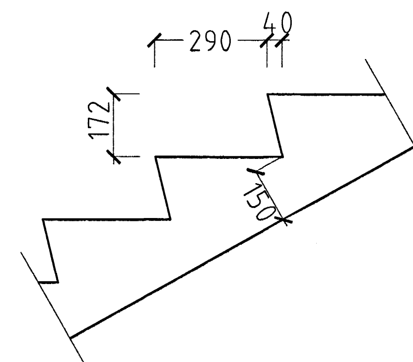
SNÍÐ Í ÞREP MKV. 1:10.
