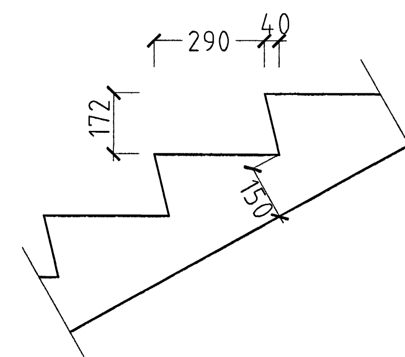
SNIB Í ÞREP MKV. 1:10.
