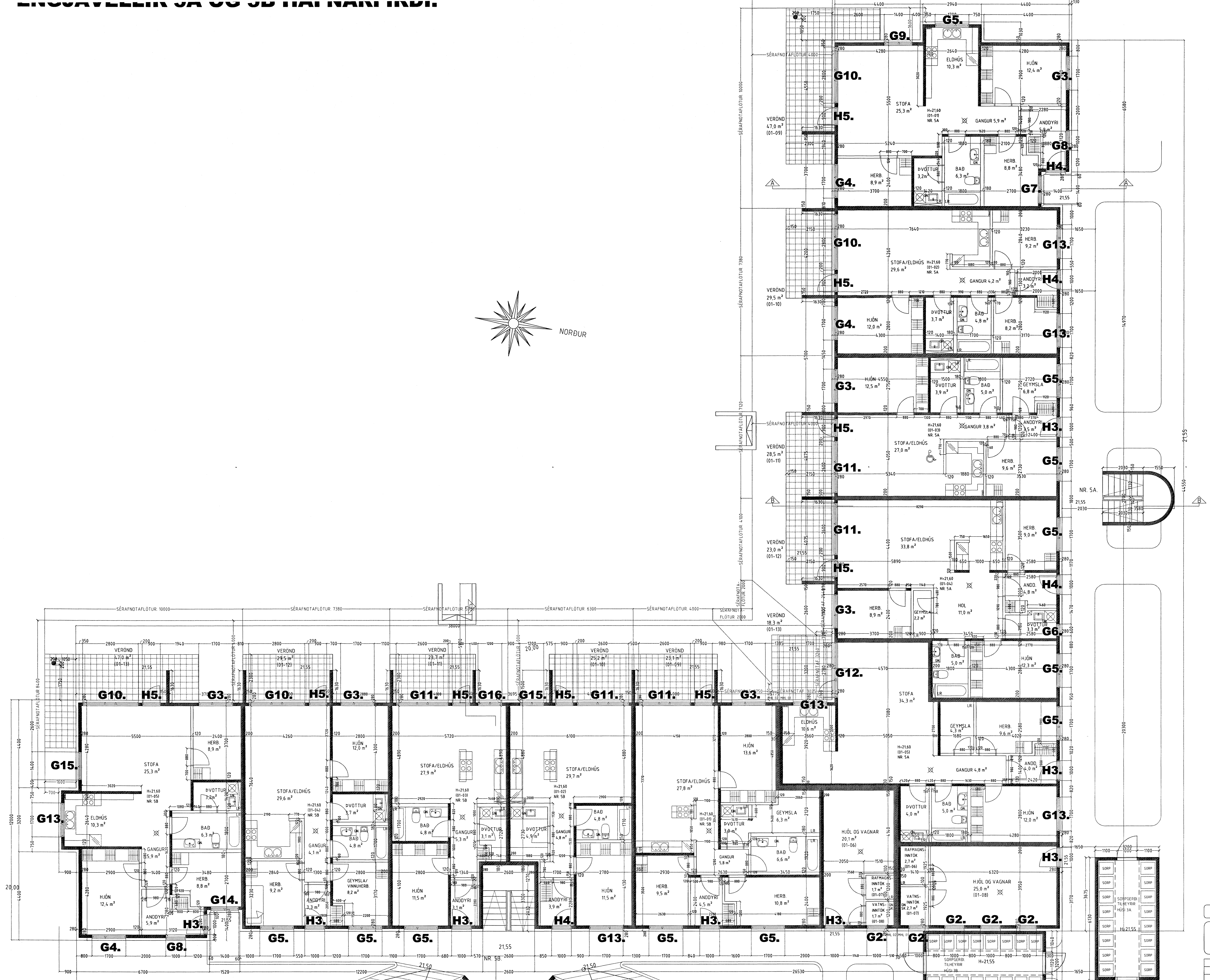
GRUNNMYND 1. HÆÐ MKV. 1:60.
