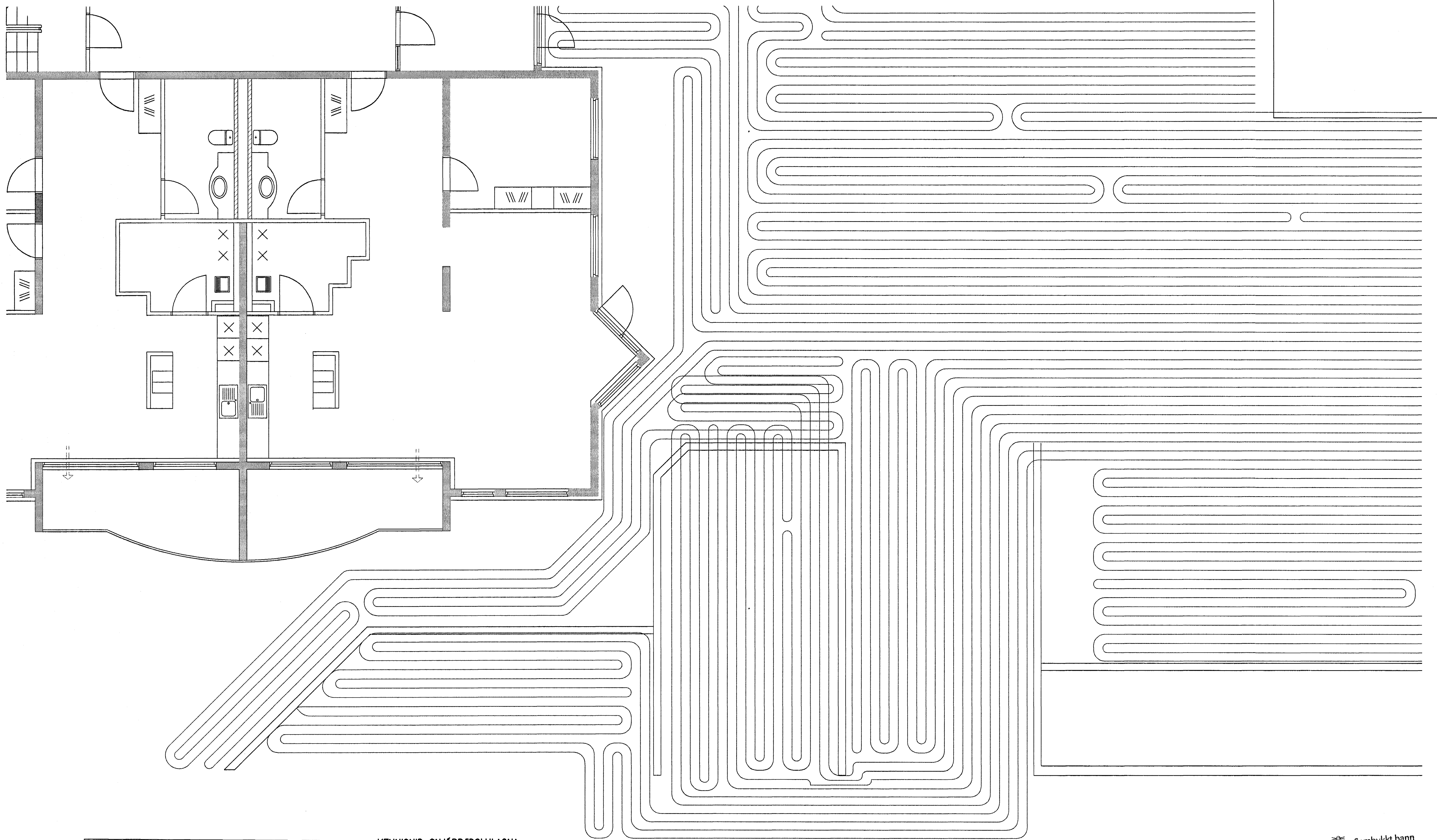
KENNISNIÐ-SNJÓBRÆDSLULAGNA 1:10
