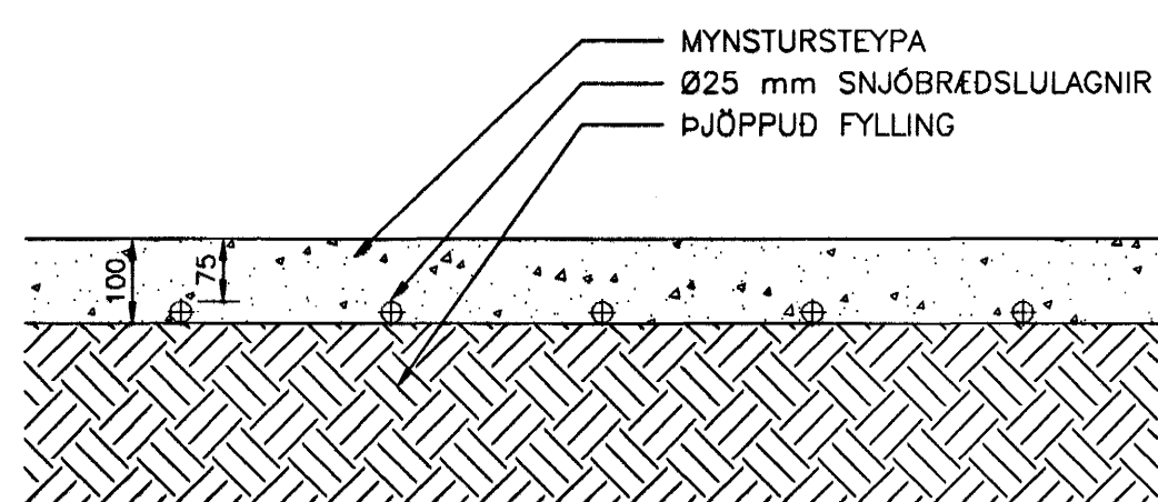
KENNISNIÐ-SNJÓBR. / MYNSTURSTEYPU 1:10
