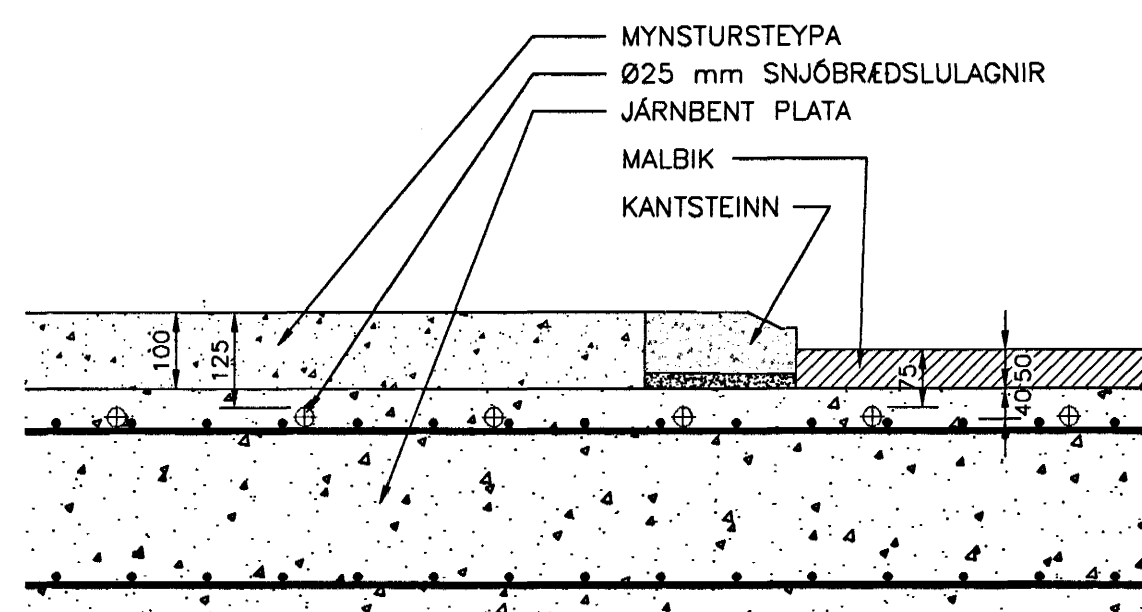
KENNISNIÐ-SNJÓBRÆDSLULAGNA 1:10
